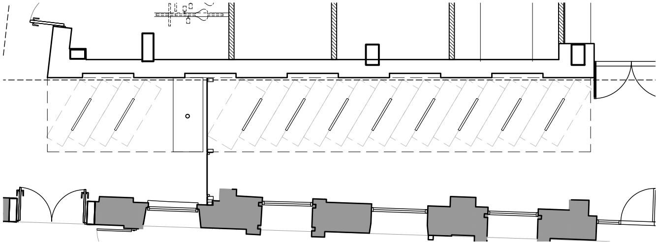
PLAN - 1:100
