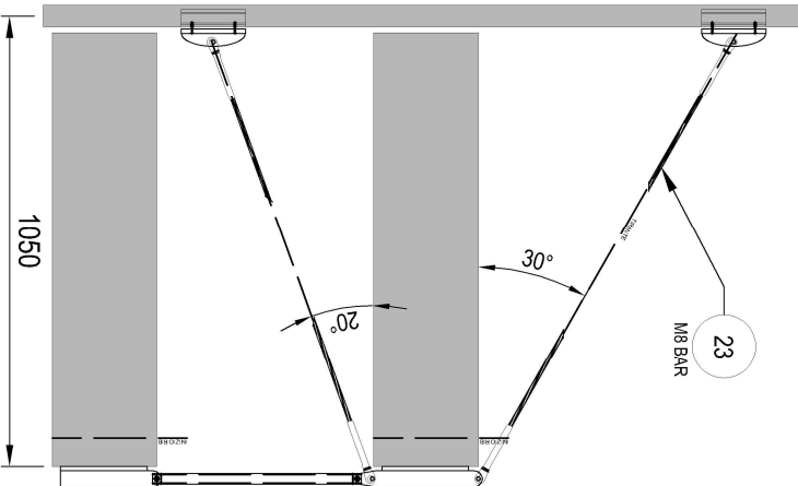
ANGLES - 1:20
