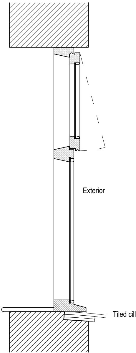
Section A-A
