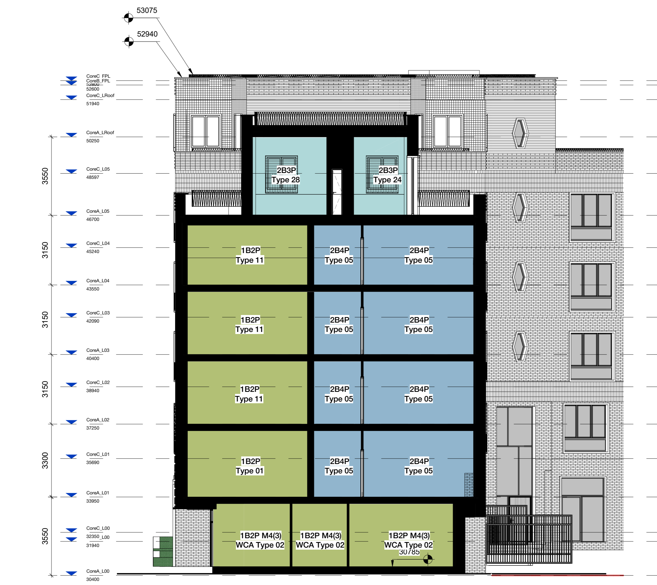
2 Section B-B 1 : 100
