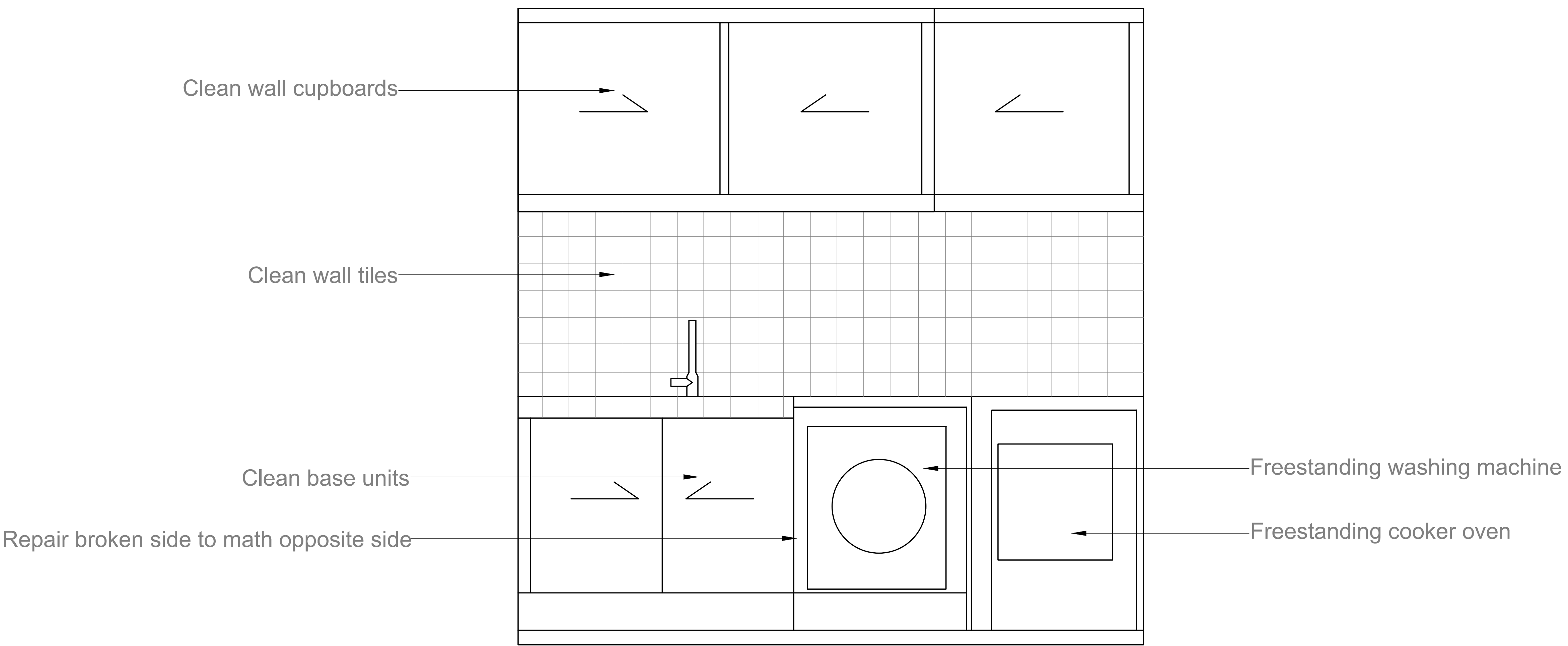
01 Section 01 1:10
