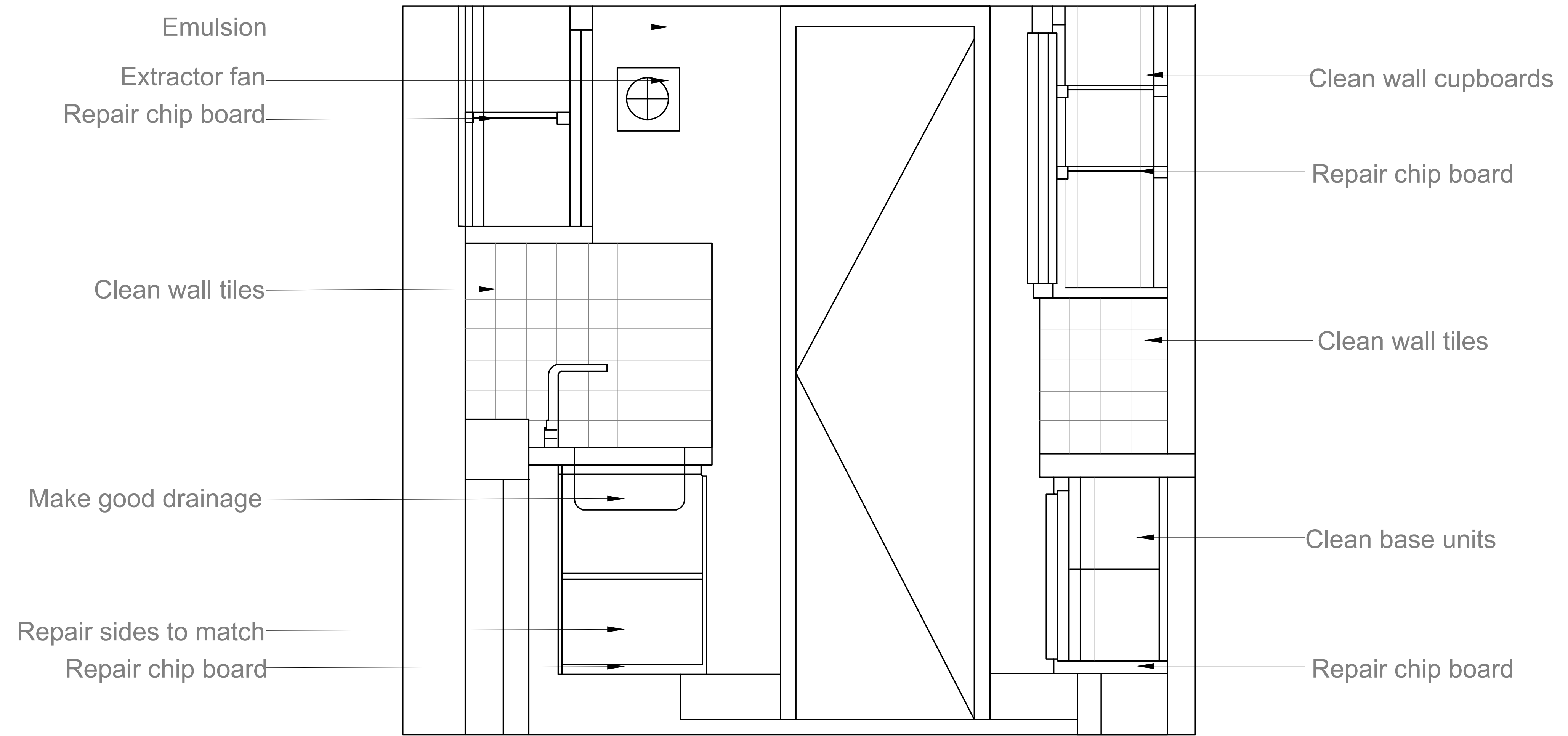
02 Section 02 1:10
