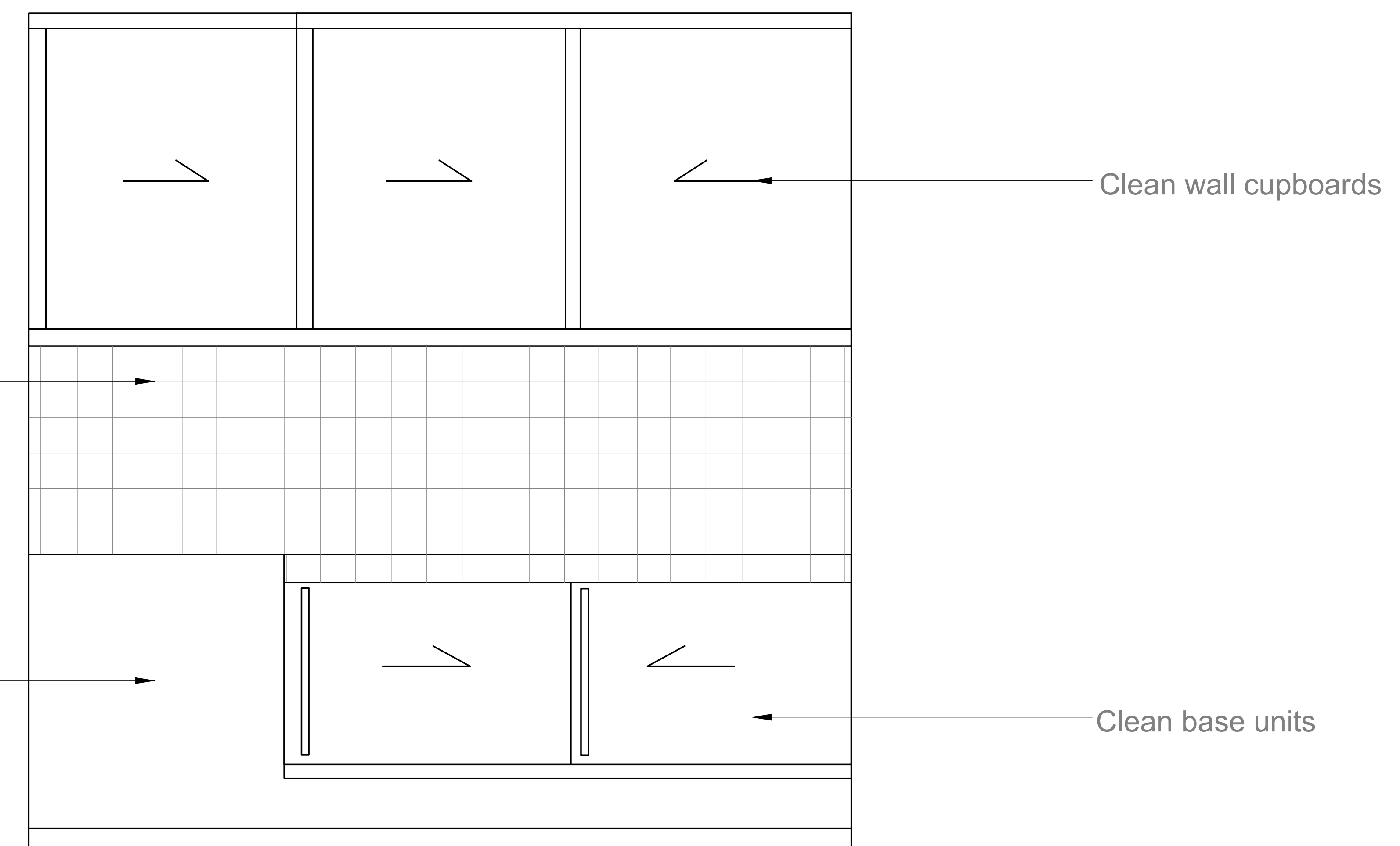
03 Section 03 1:10
