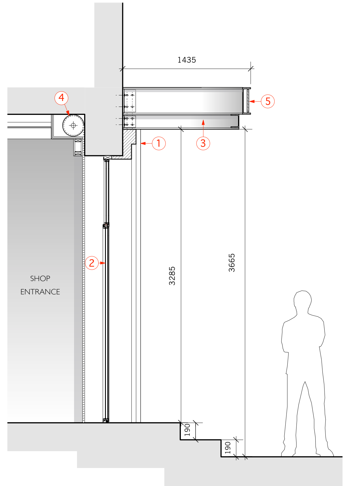
SECTION A-A 1:25
