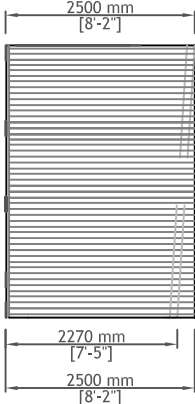
Right Elevation
