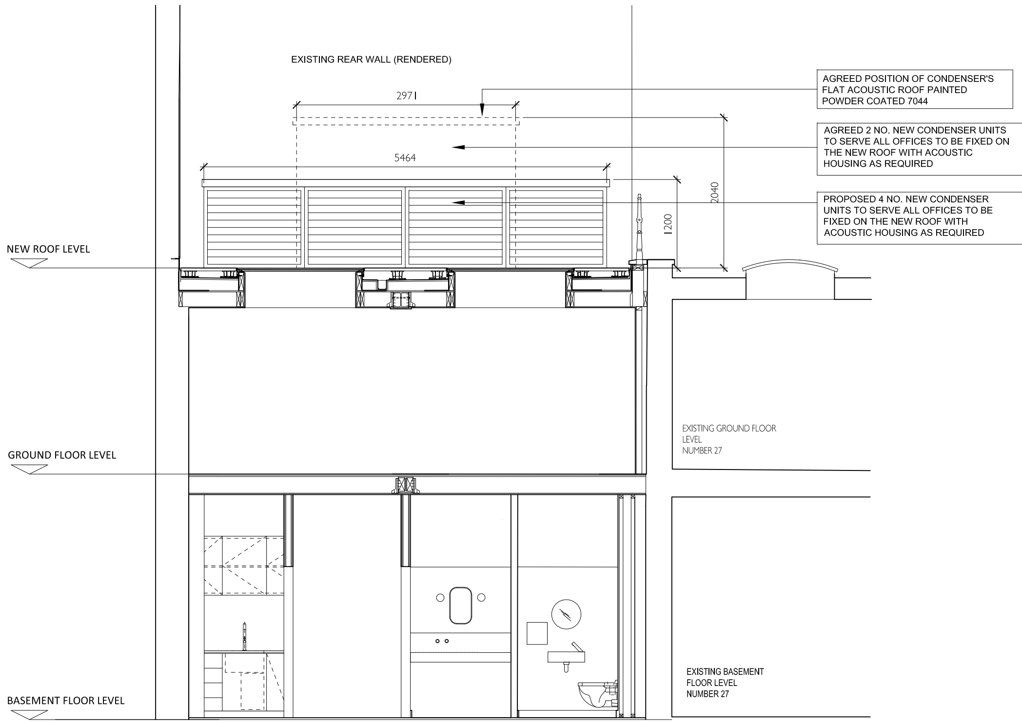
SECTION DD
