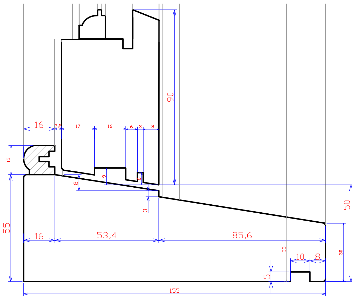
1 Sill Scale 1:1
