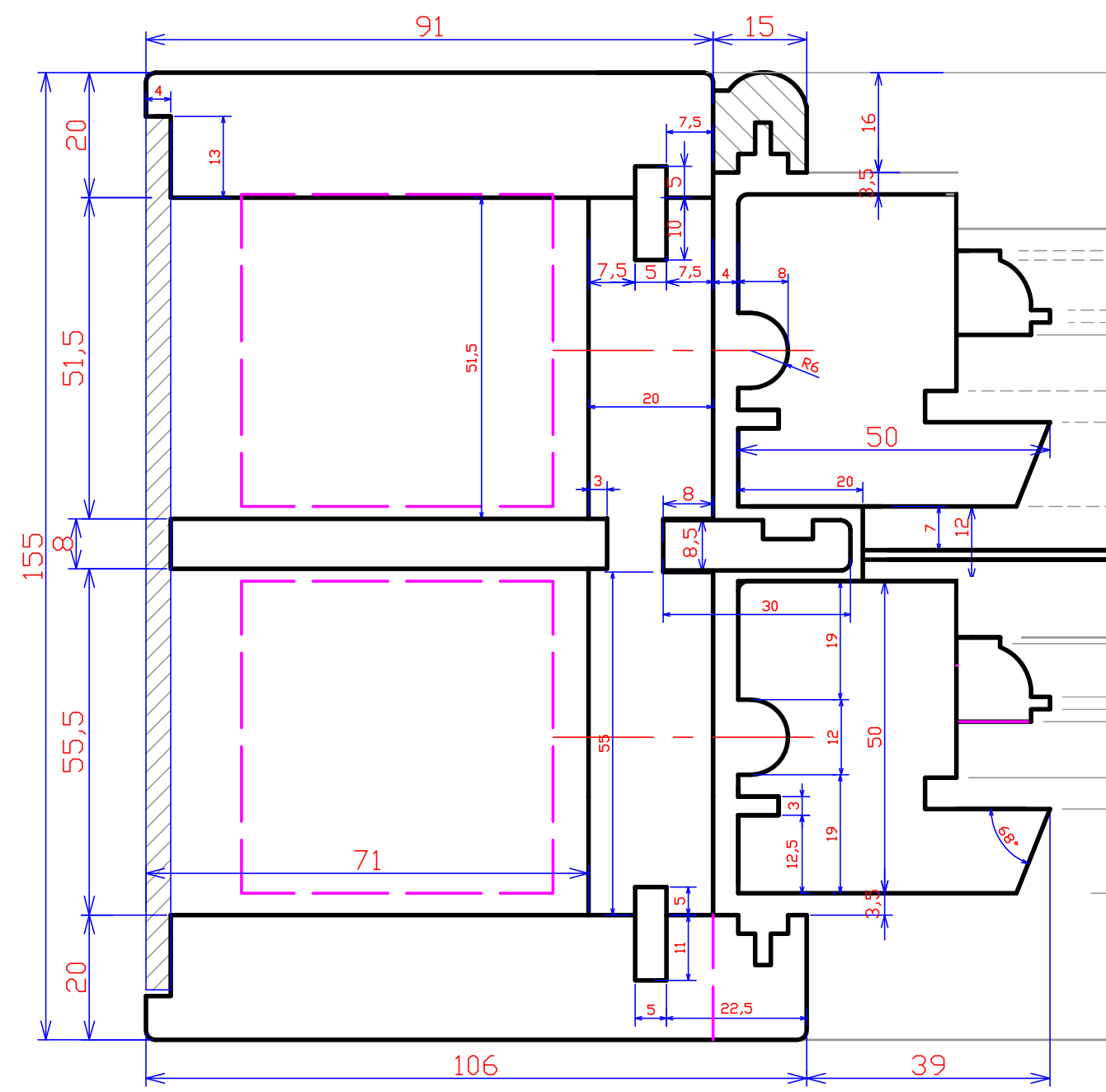
4 Jamb Scale 1:1
