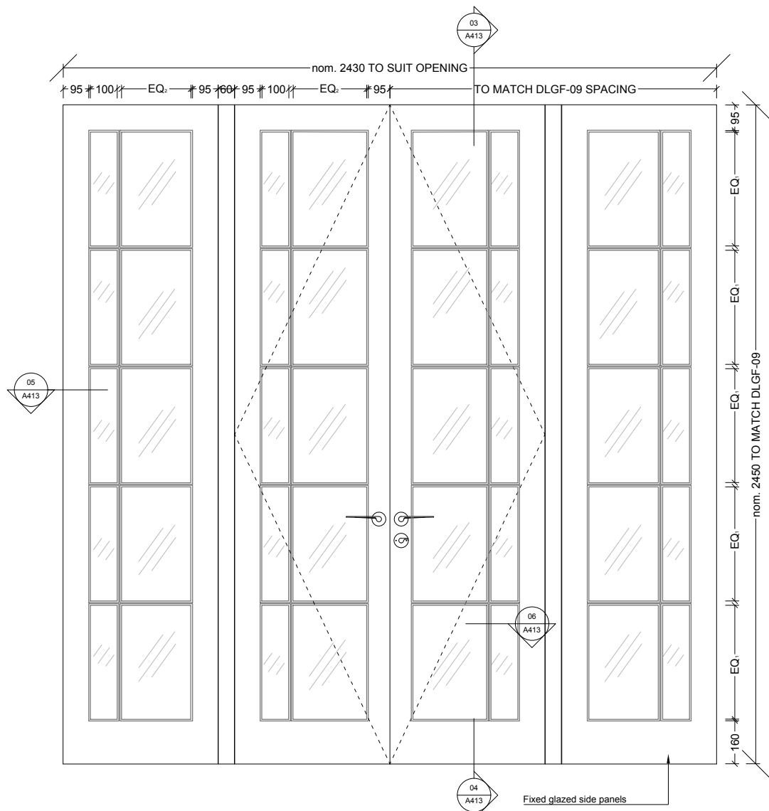
01 DOOR TYPE 2E - PROPOSED ELEVATION 1:20@A3, 1:10@A1
