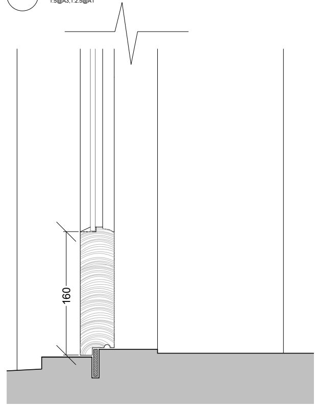
04 DOOR TYPE 2E - THRESHOLD DETAIL 1:5@A3, 1:2.5@A1
