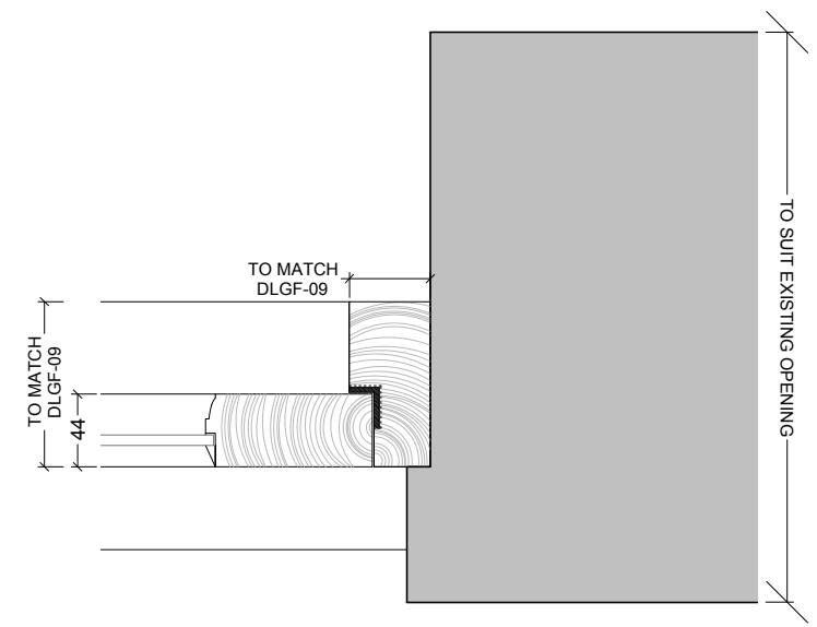
05 DOOR TYPE 2E - JAMB DETAIL 1:5@A3, 1:2.5@A1
