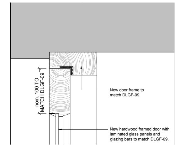
03 DOOR TYPE 2E - HEAD DETAIL 1:5@A3, 1:2.5@A1
