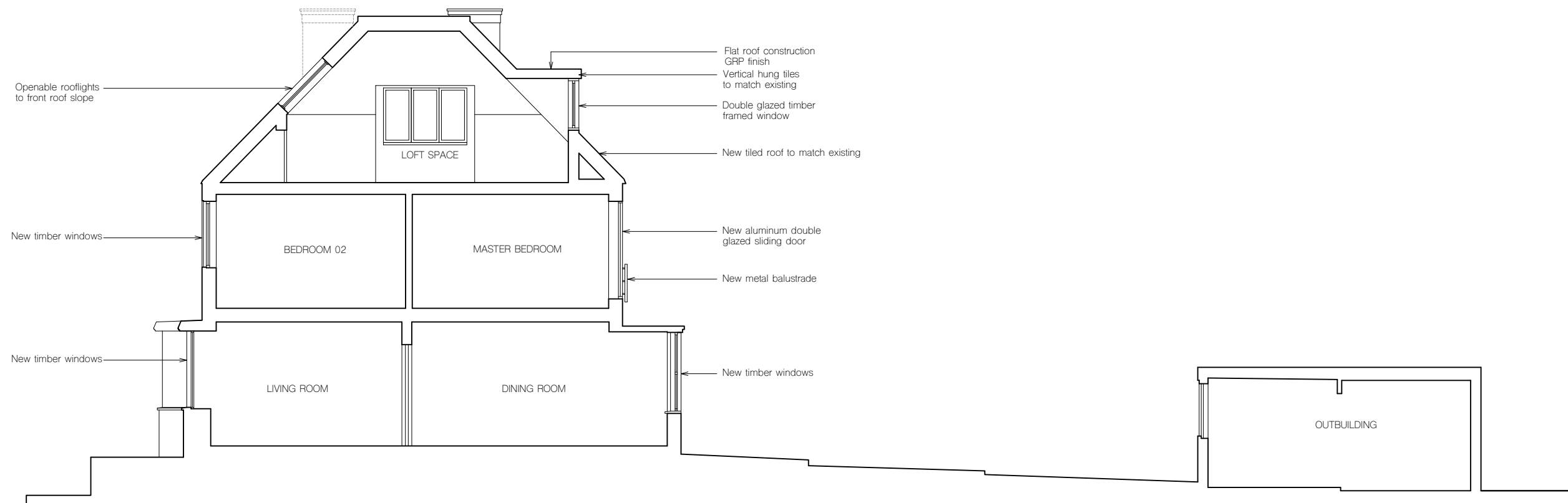
2 longitudinal section
