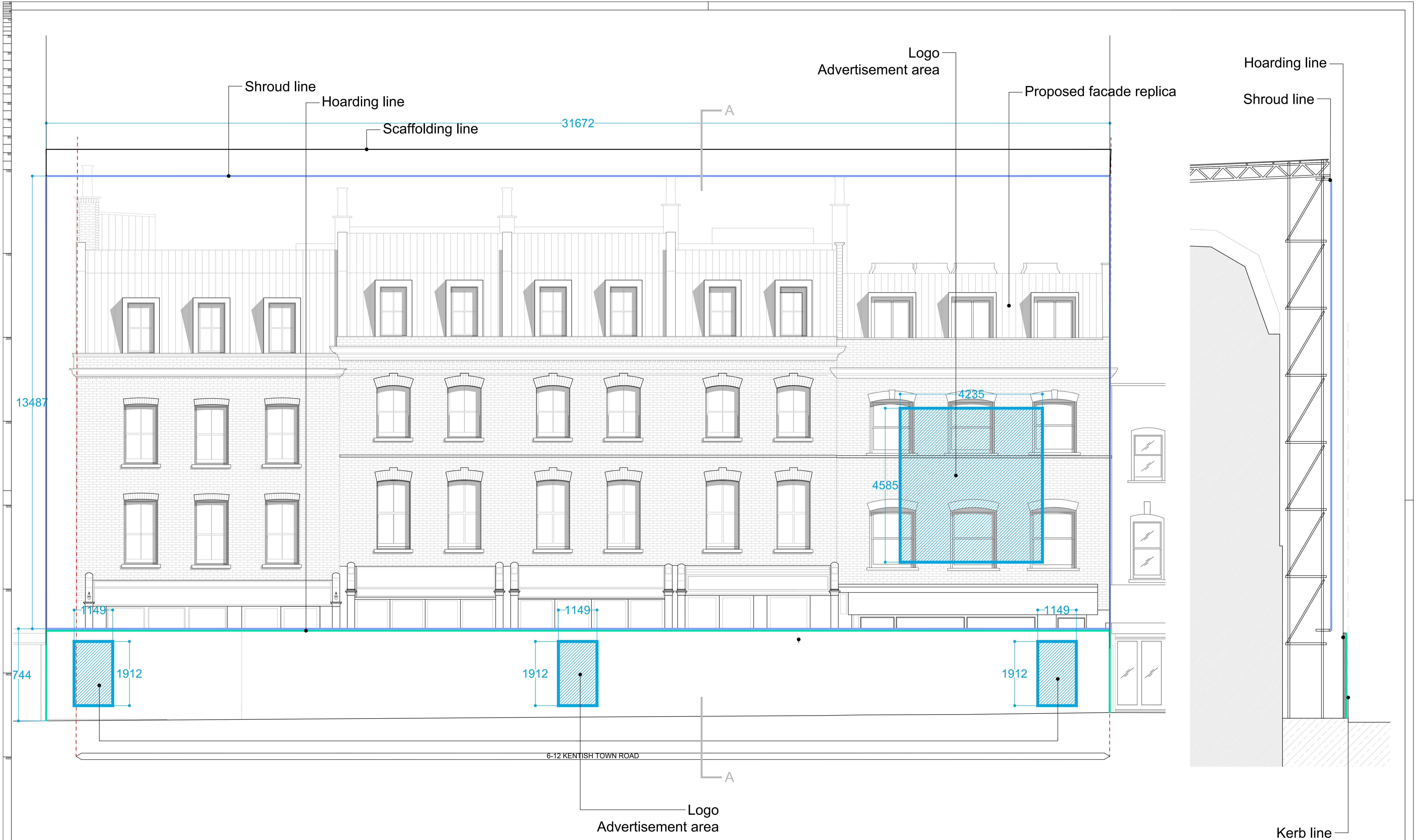
00_Front elevation
