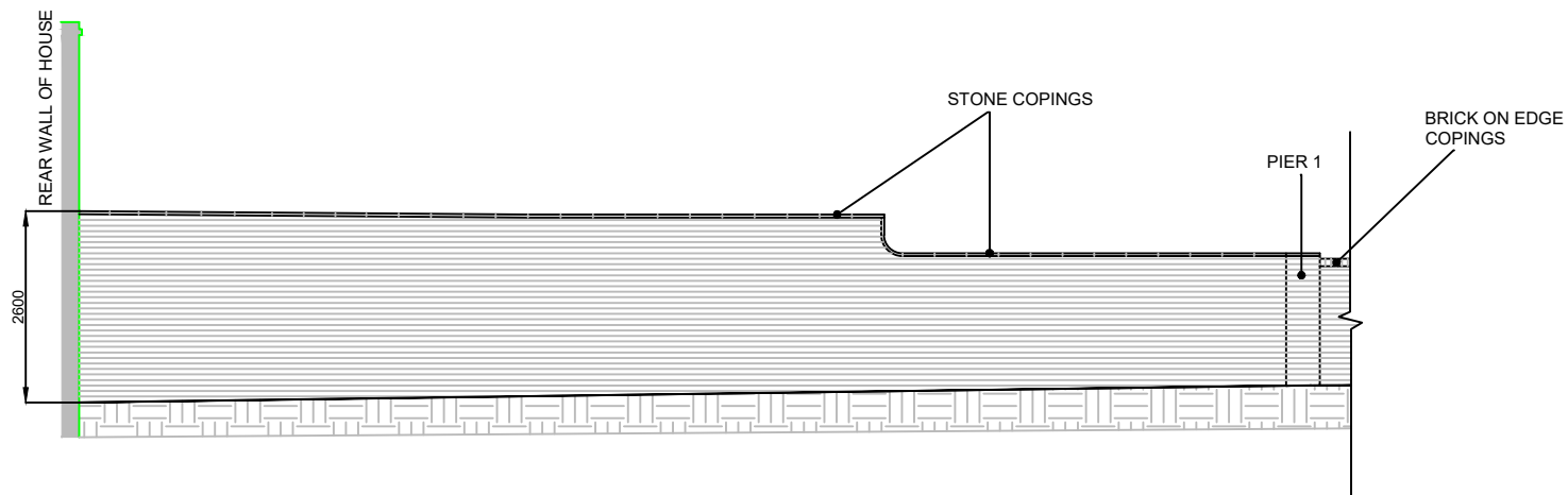
ELEVATION
