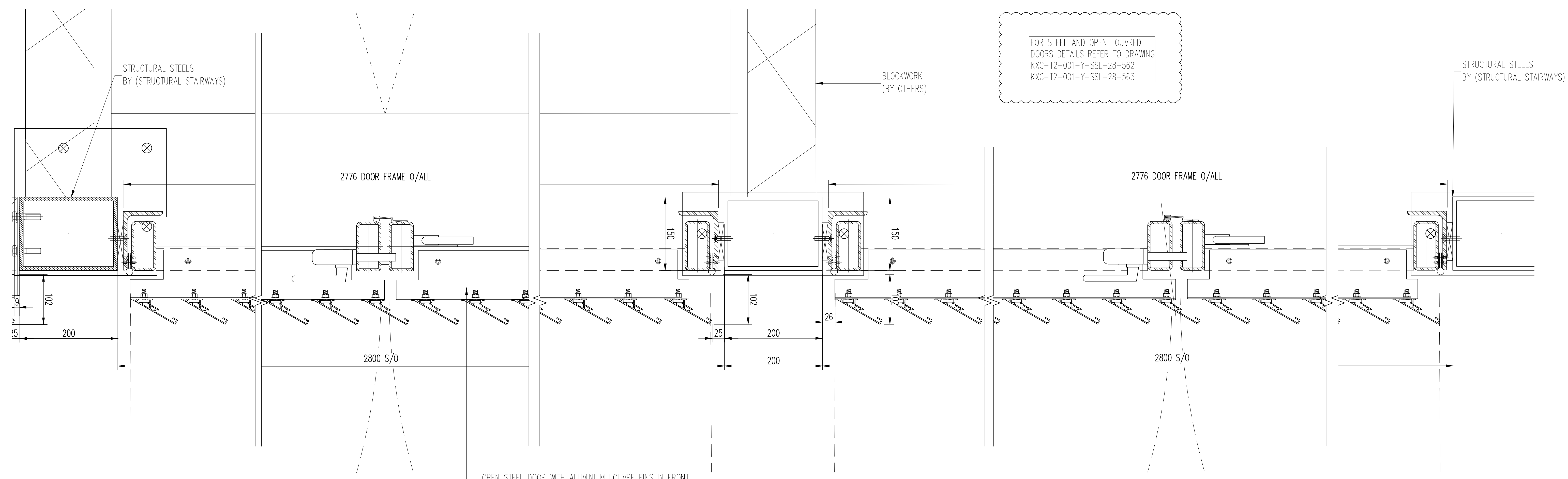
01 DOOR 00-C07-ED02 HORIZONTAL SECTION 1:4
