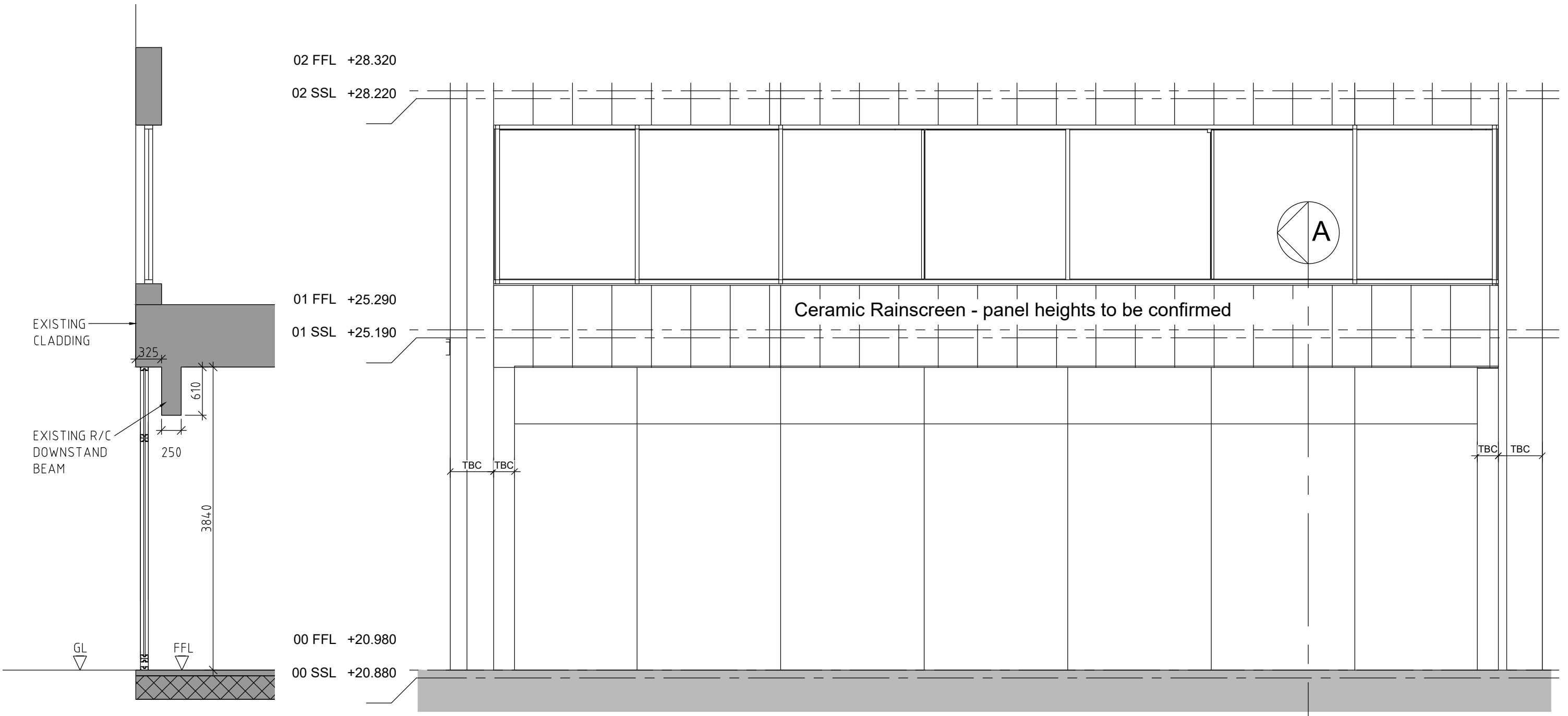
SECTION A-A
