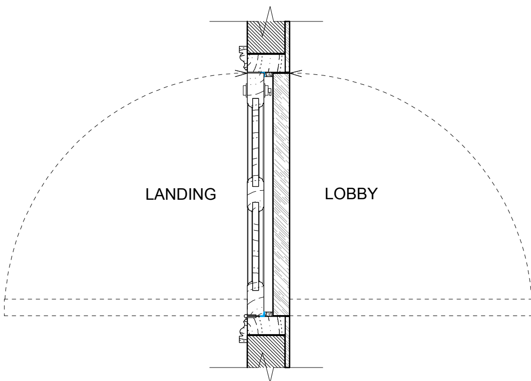
4 503 Lobby Door Plan Scale: 1:10 FD.30.S
