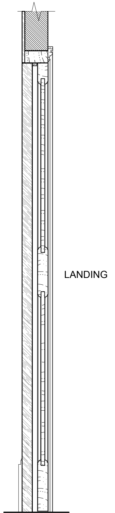
3 503 Door Section Scale: 1:10
