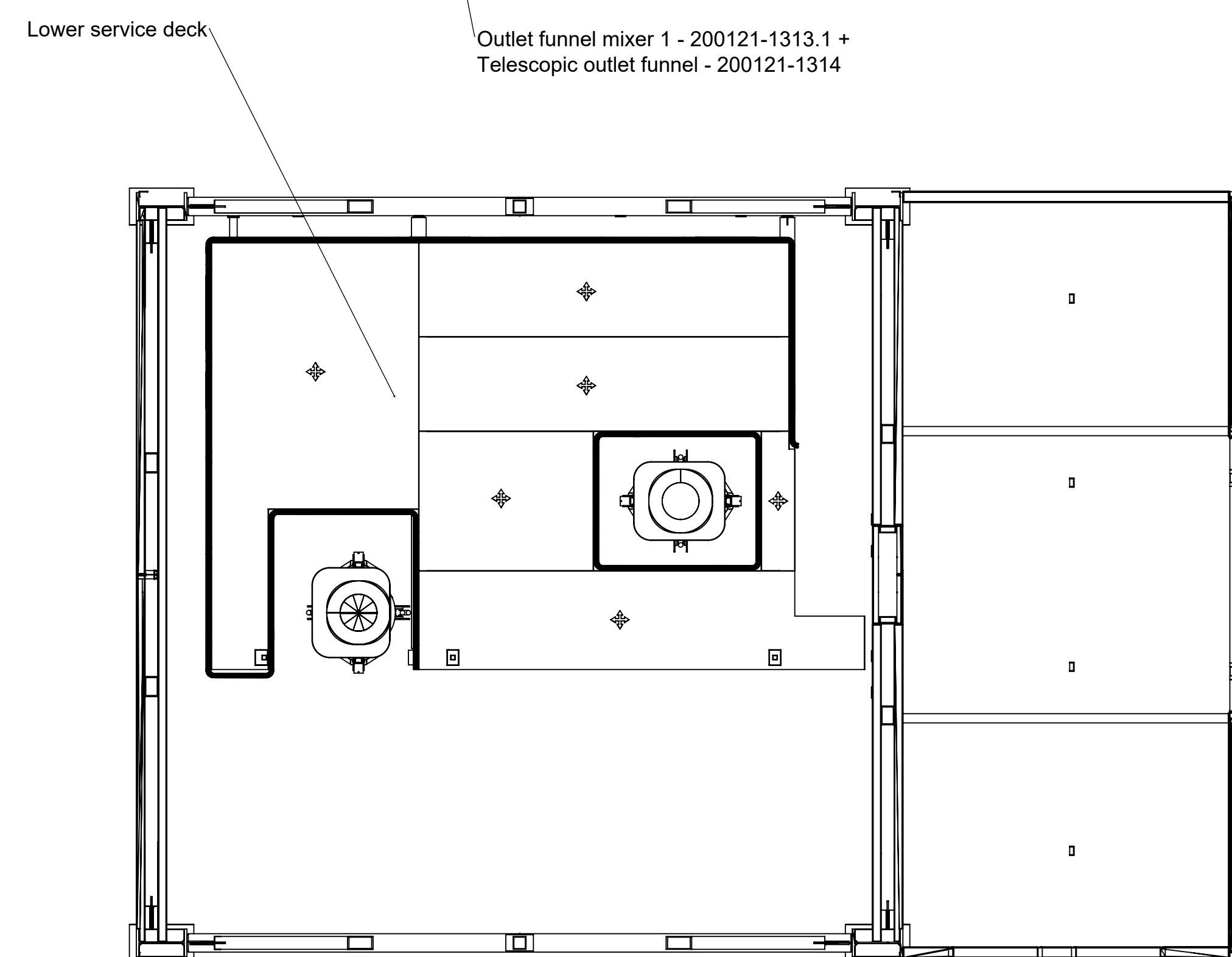
SECTION A-A
