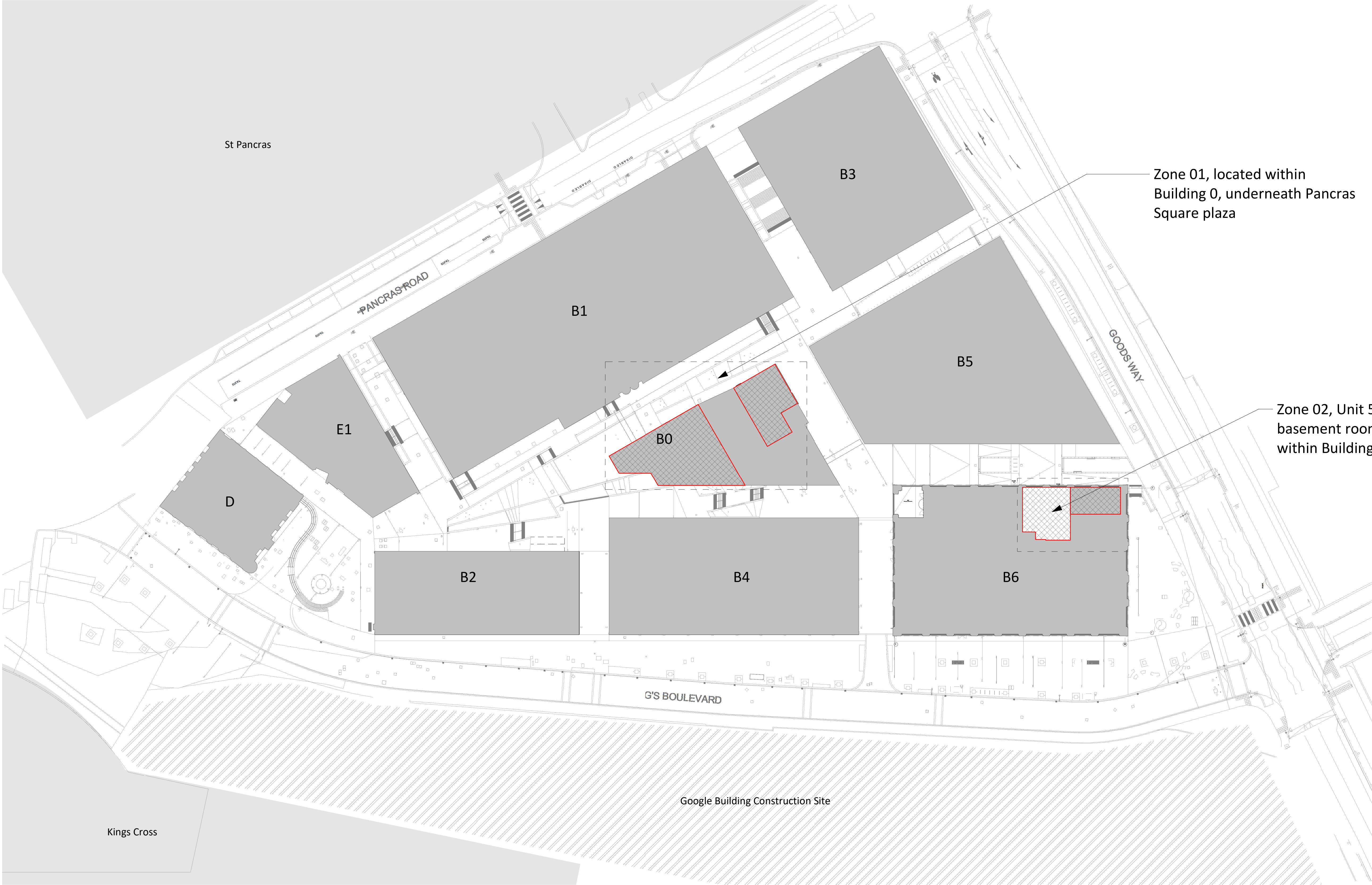
Site Plan 1 : 500
