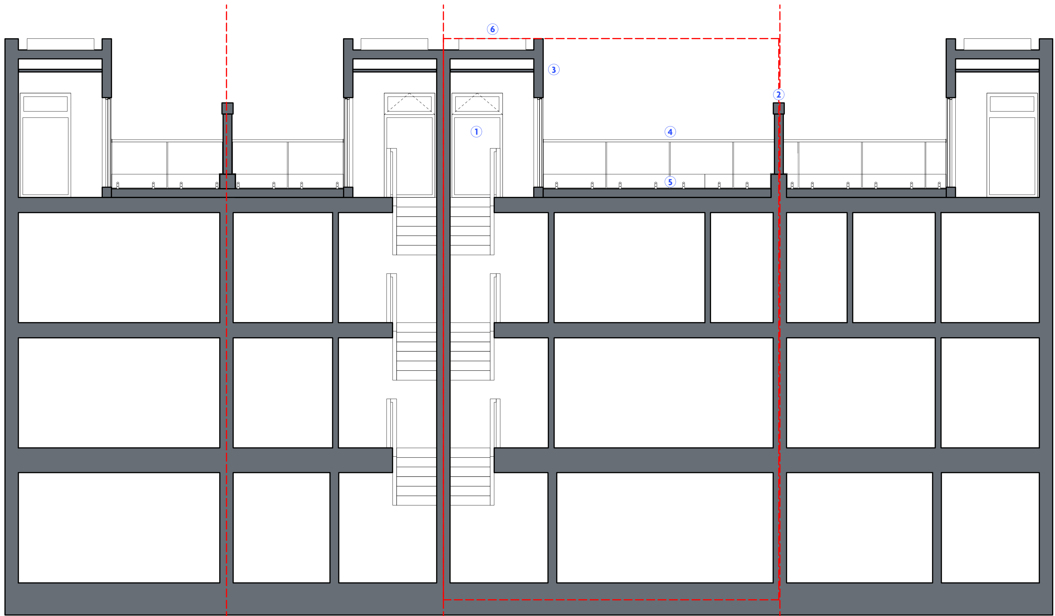
2 Existing Section C-C Scale: 1:50
