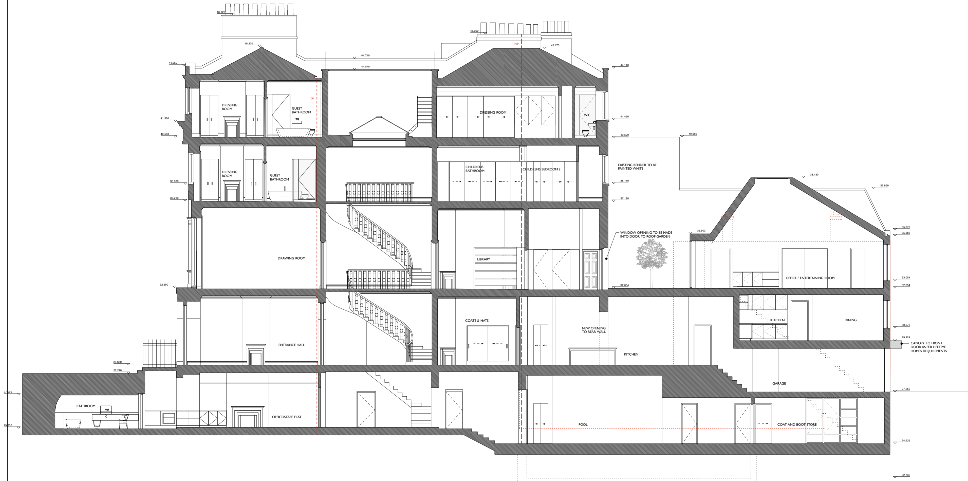
SECTION DD
