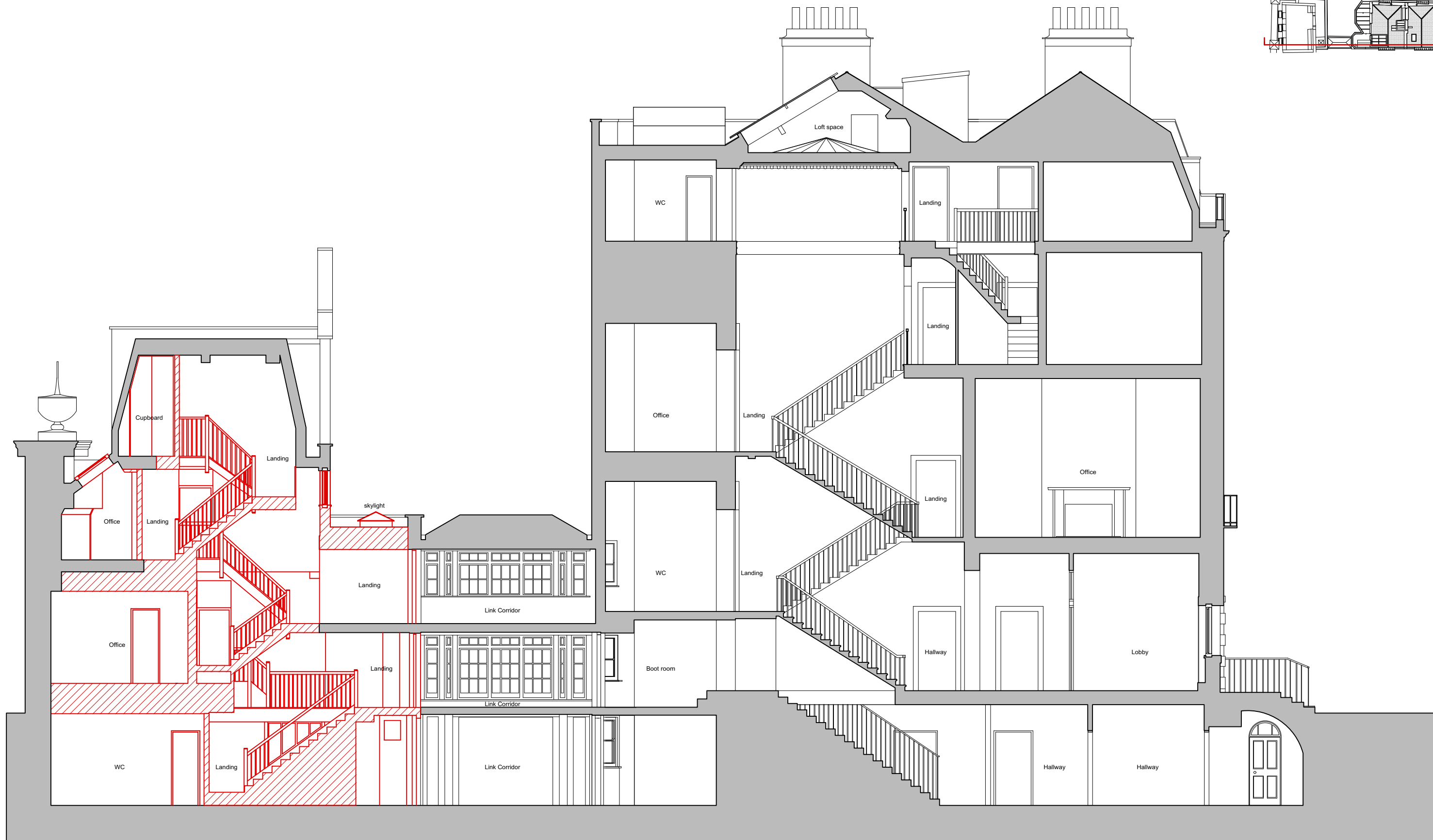
1 Demolition Section AA Scale: 1:100 @ A3
