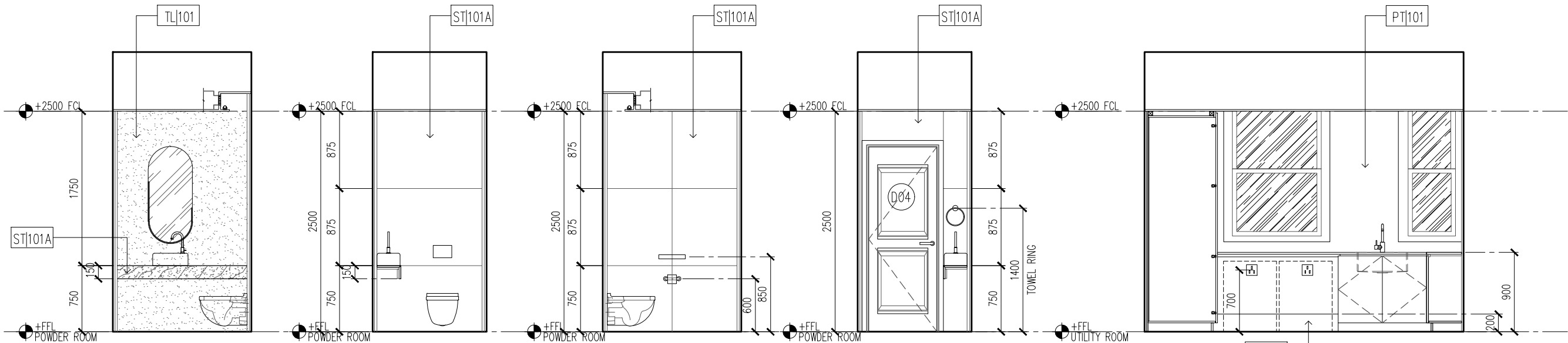
5 ELEVATION 105-E8 1:50
