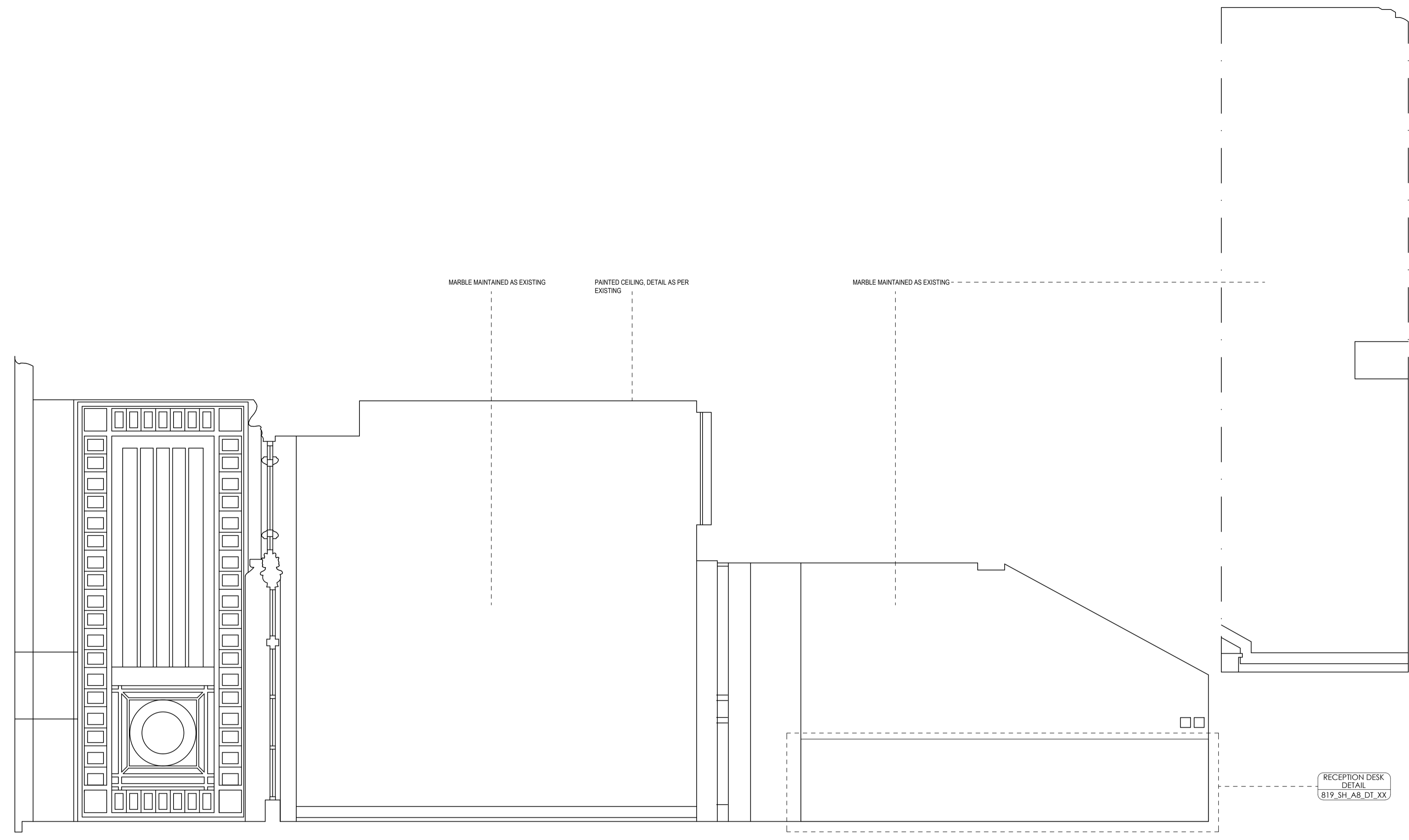
E ELEVATION SCALE: 1:25
