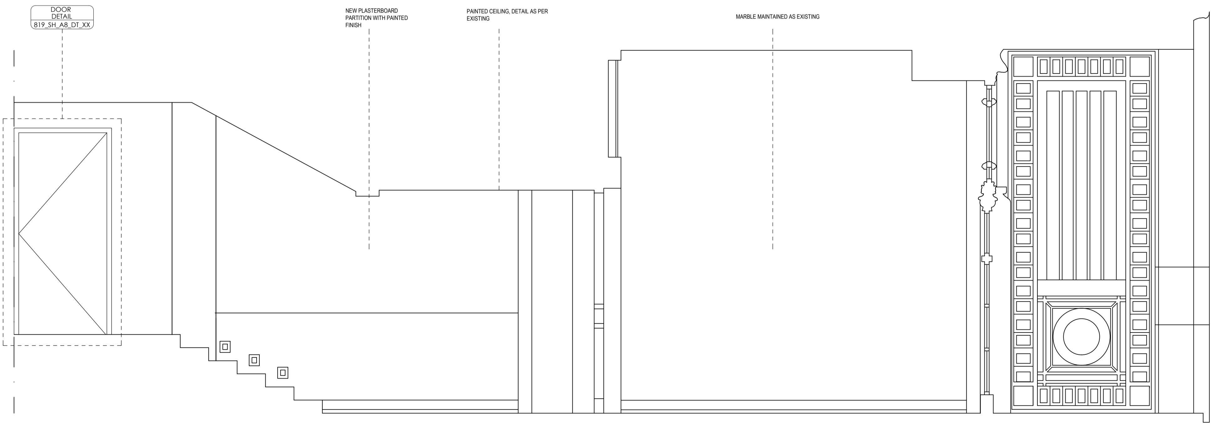
F ELEVATION SCALE: 1:25
