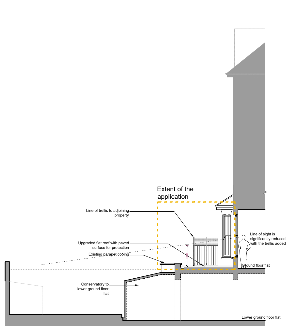
Section A-A
