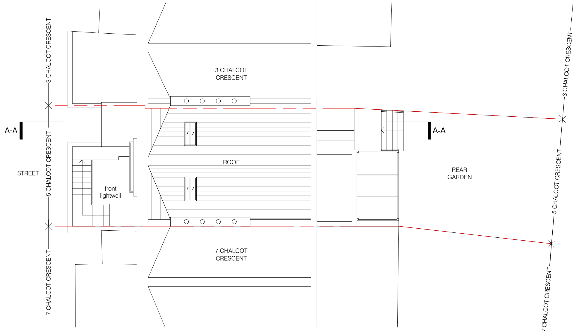
01 EXISTING SITE PLAN scale 1:100
