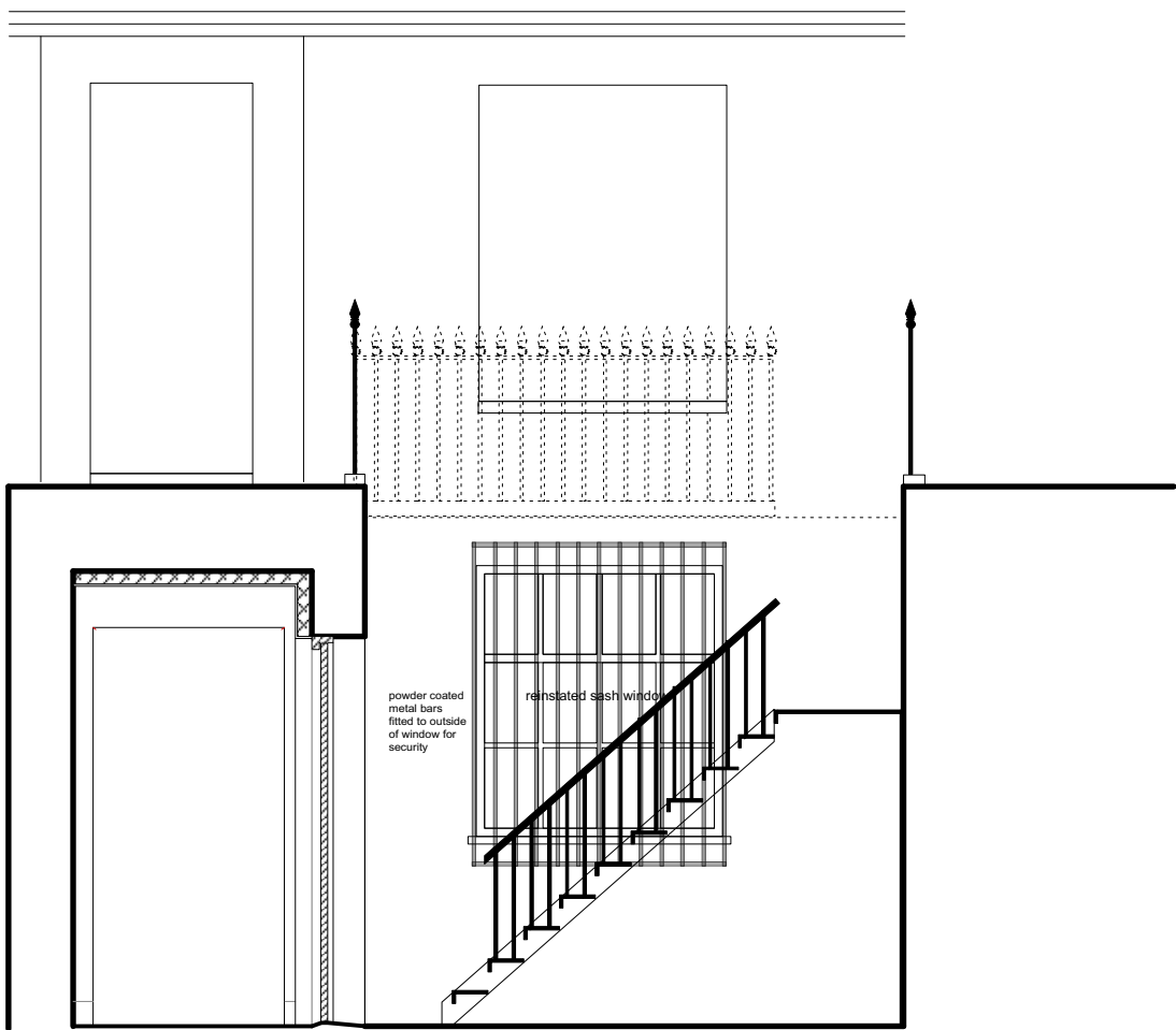
SECTION D-D
