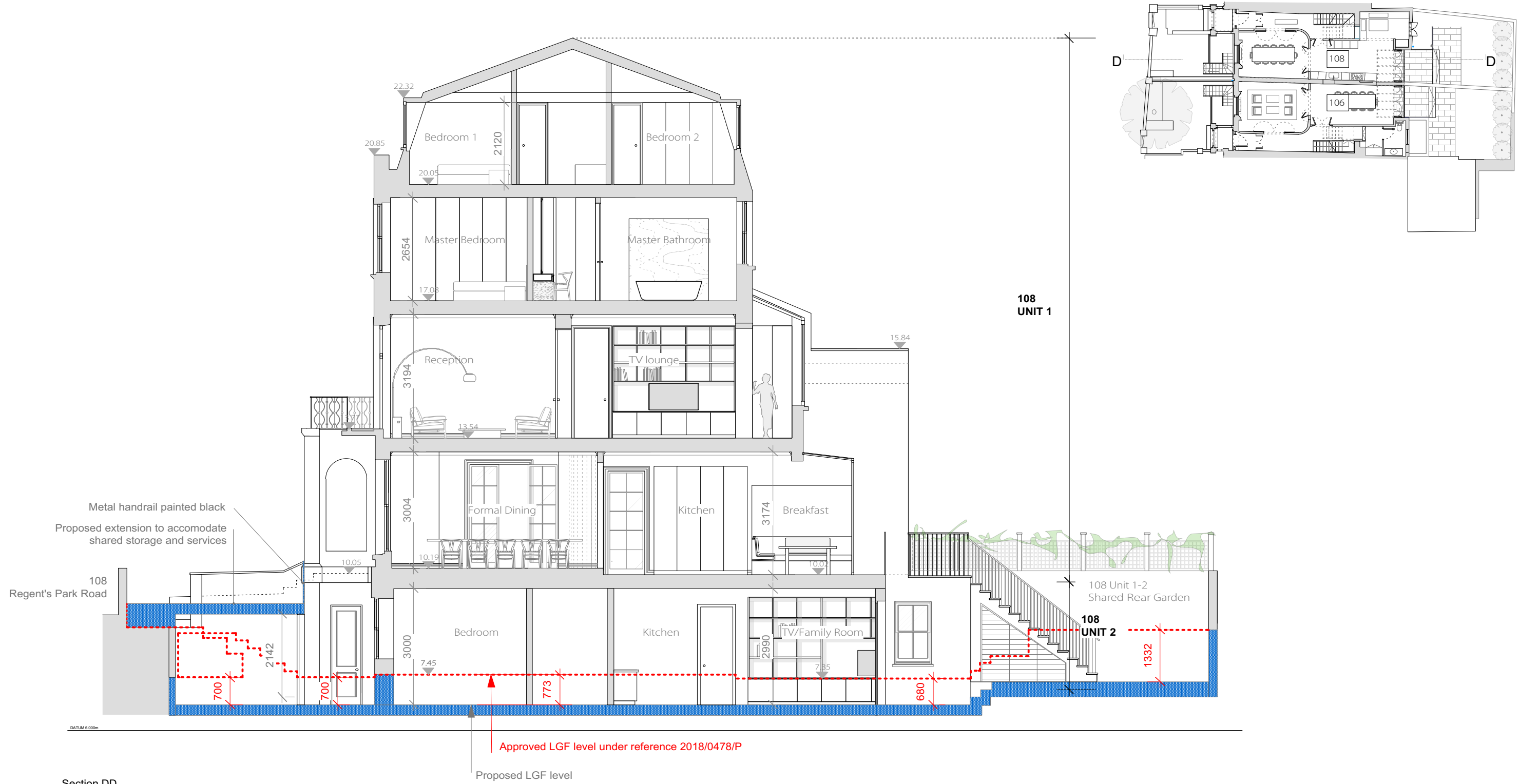
Section DD
