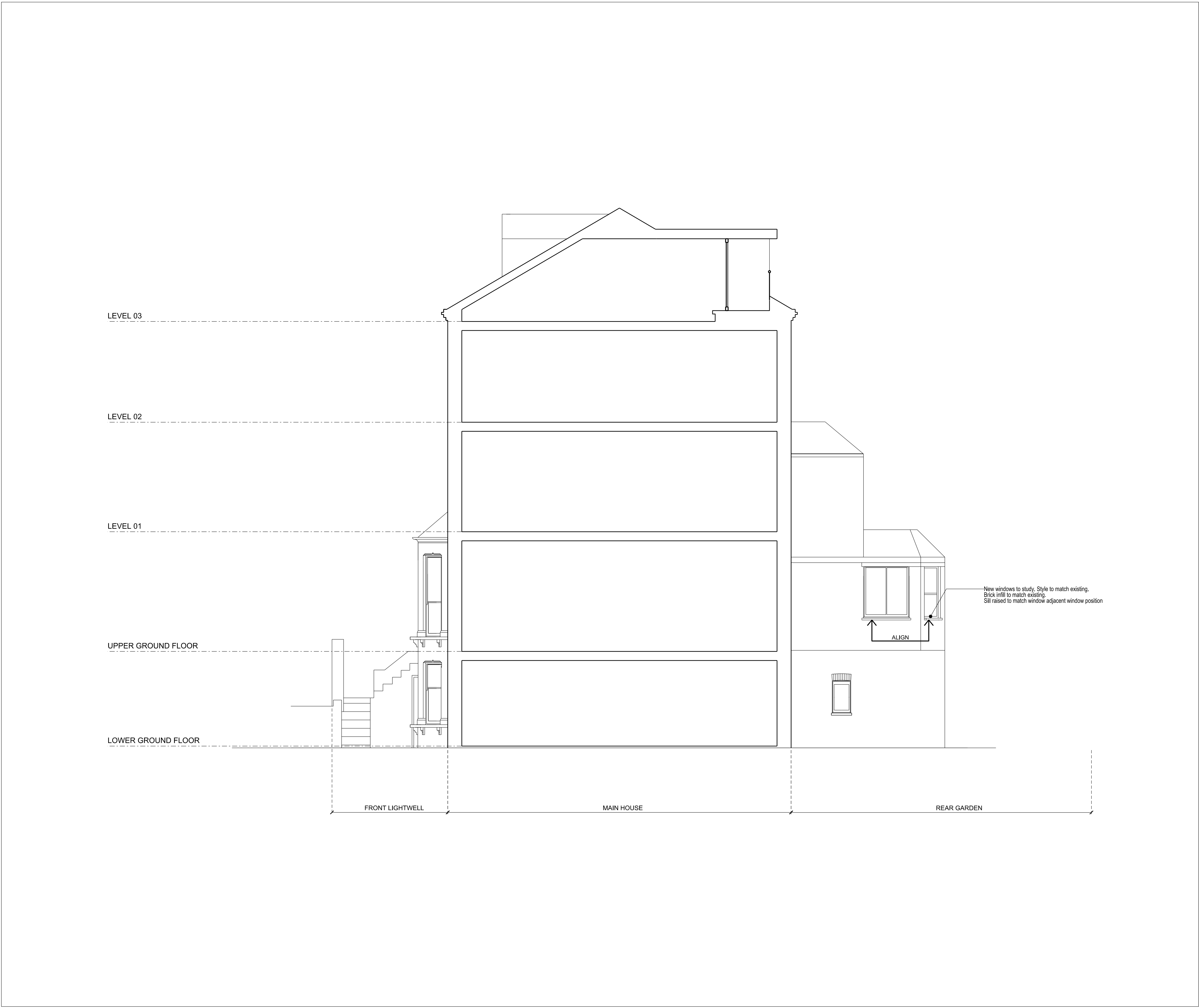
01 - SECTION
