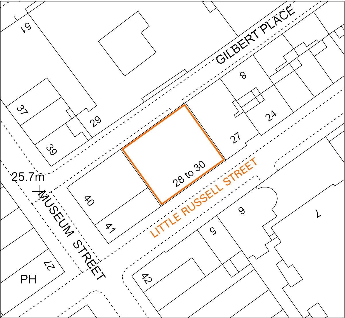
SITE PLAN 1:500
