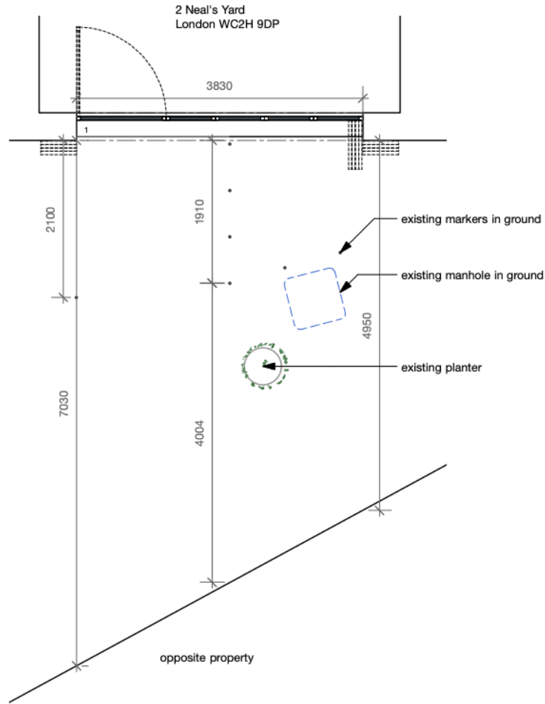
1 existing plan Scale: 1:50
