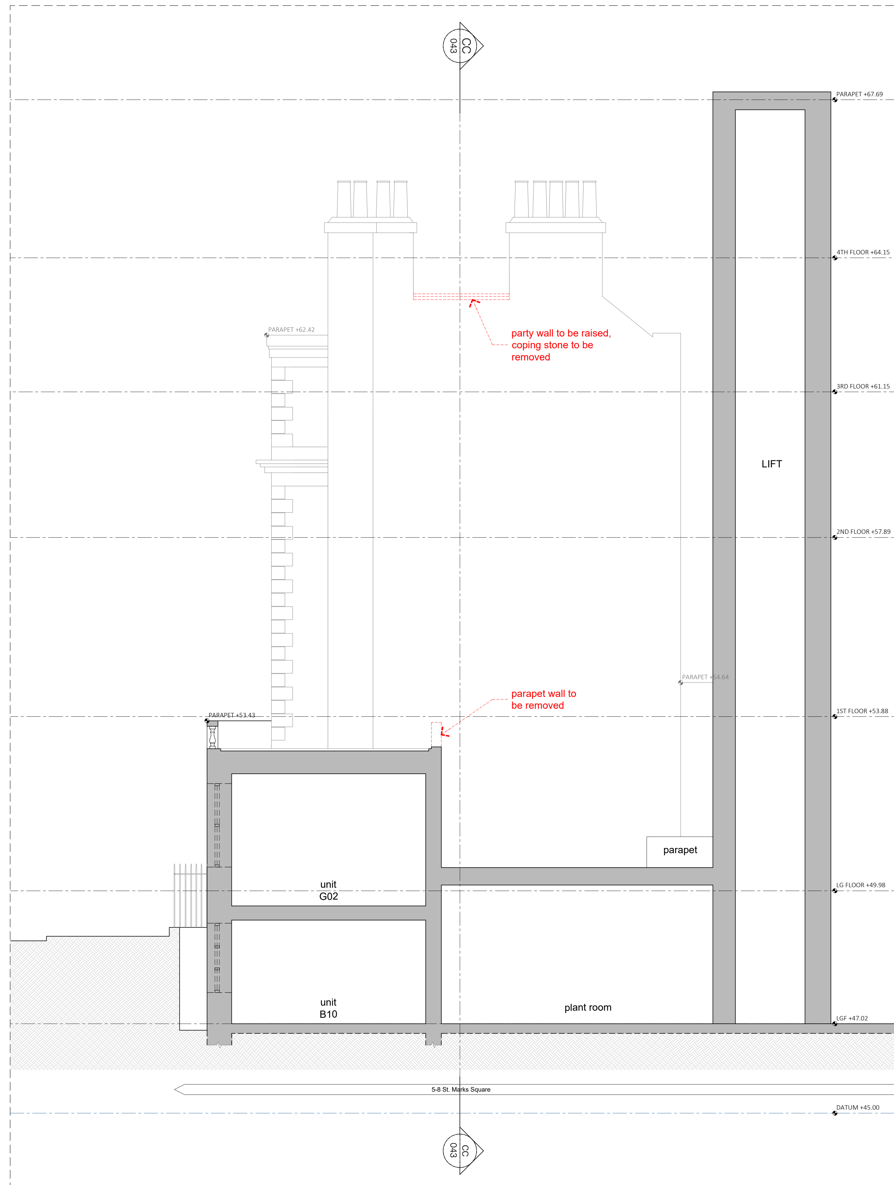
01 Existing section DD 1:50 @ A1 / 1:100 @ A3
