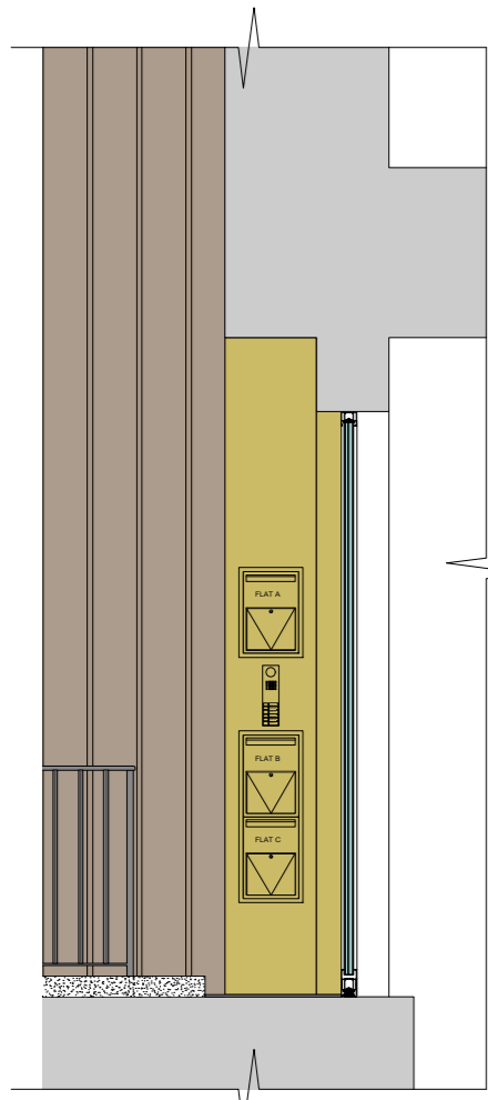
1 SECTION A-A
