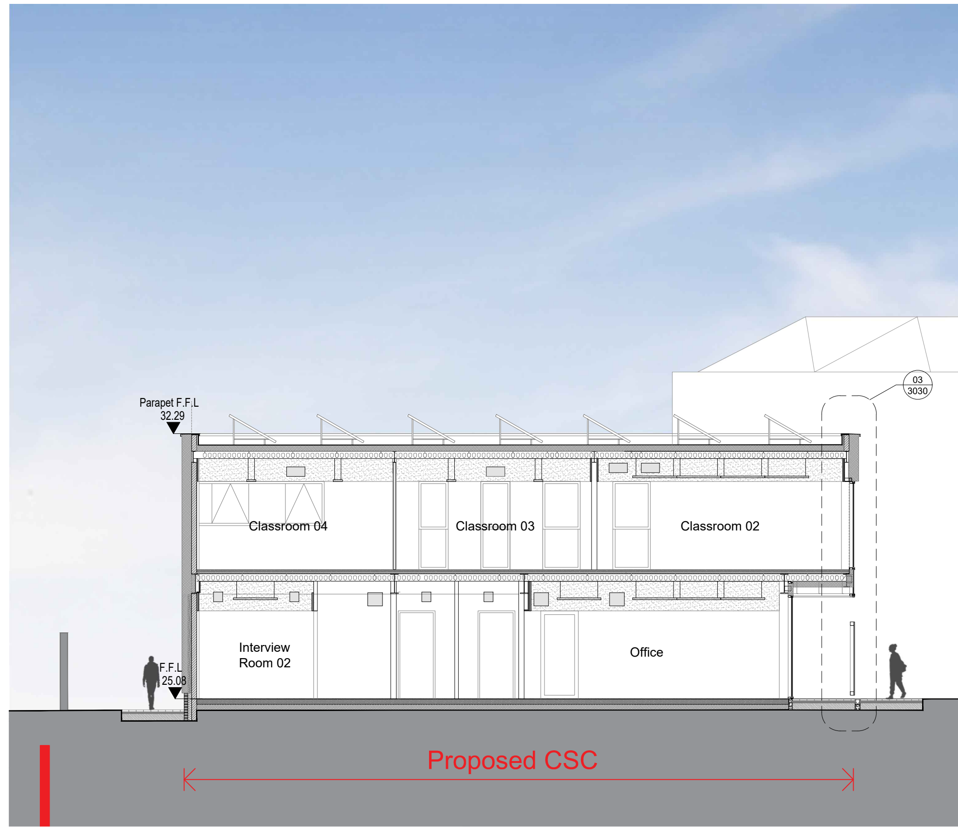
01 Section A-A
