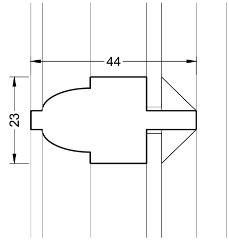
Glazing Bar 1:1
