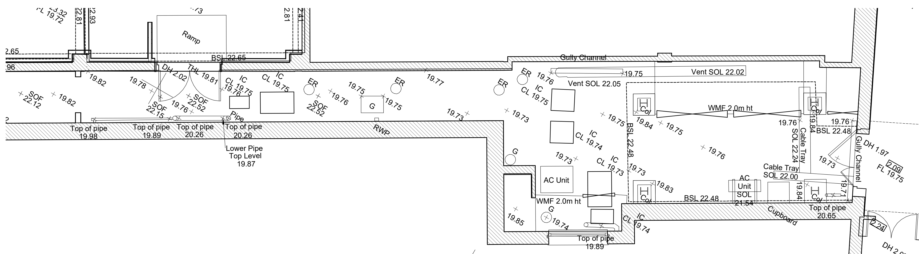
Existing Dirty Corridor 1 : 50
