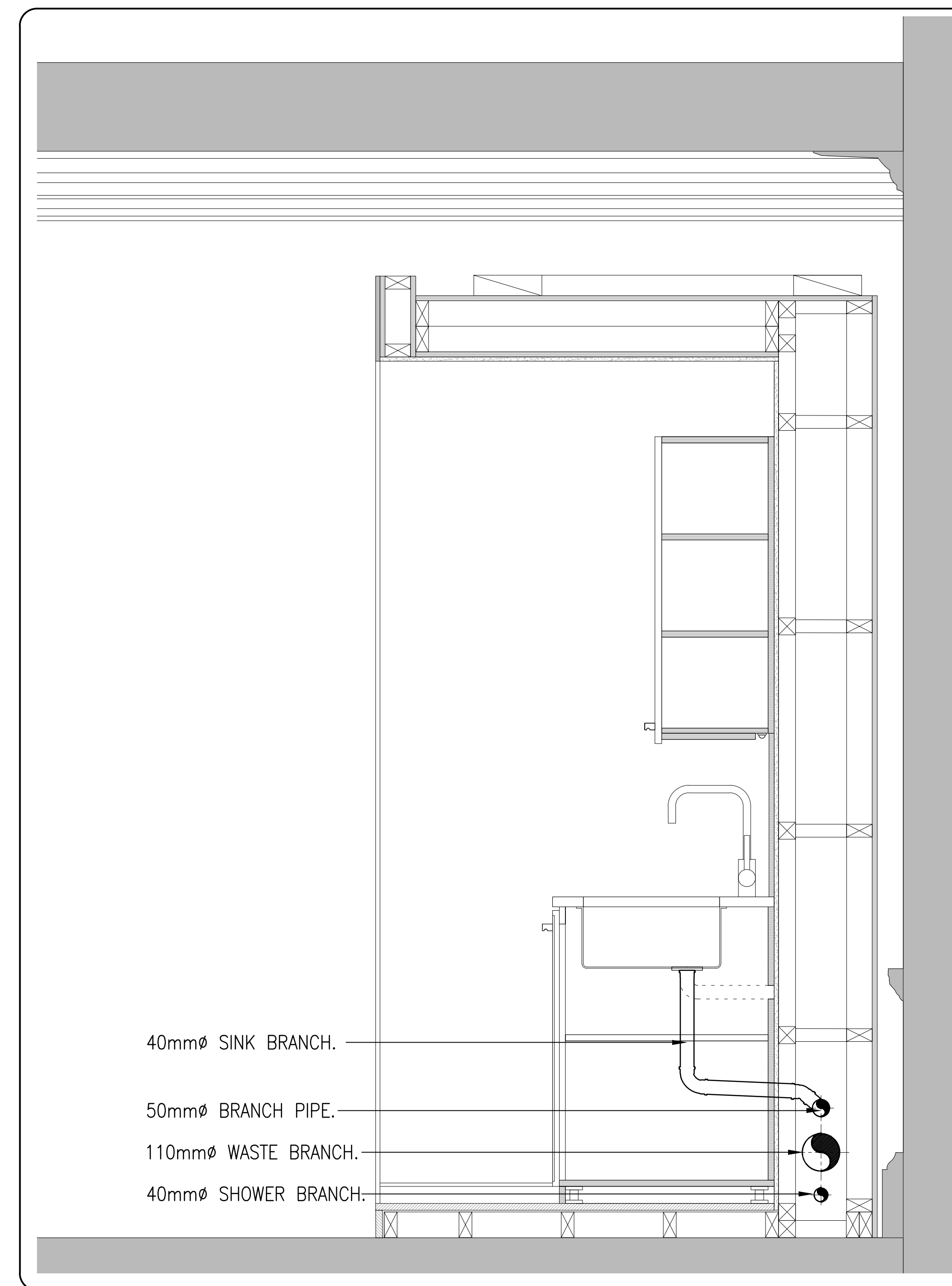
ELEVATION
