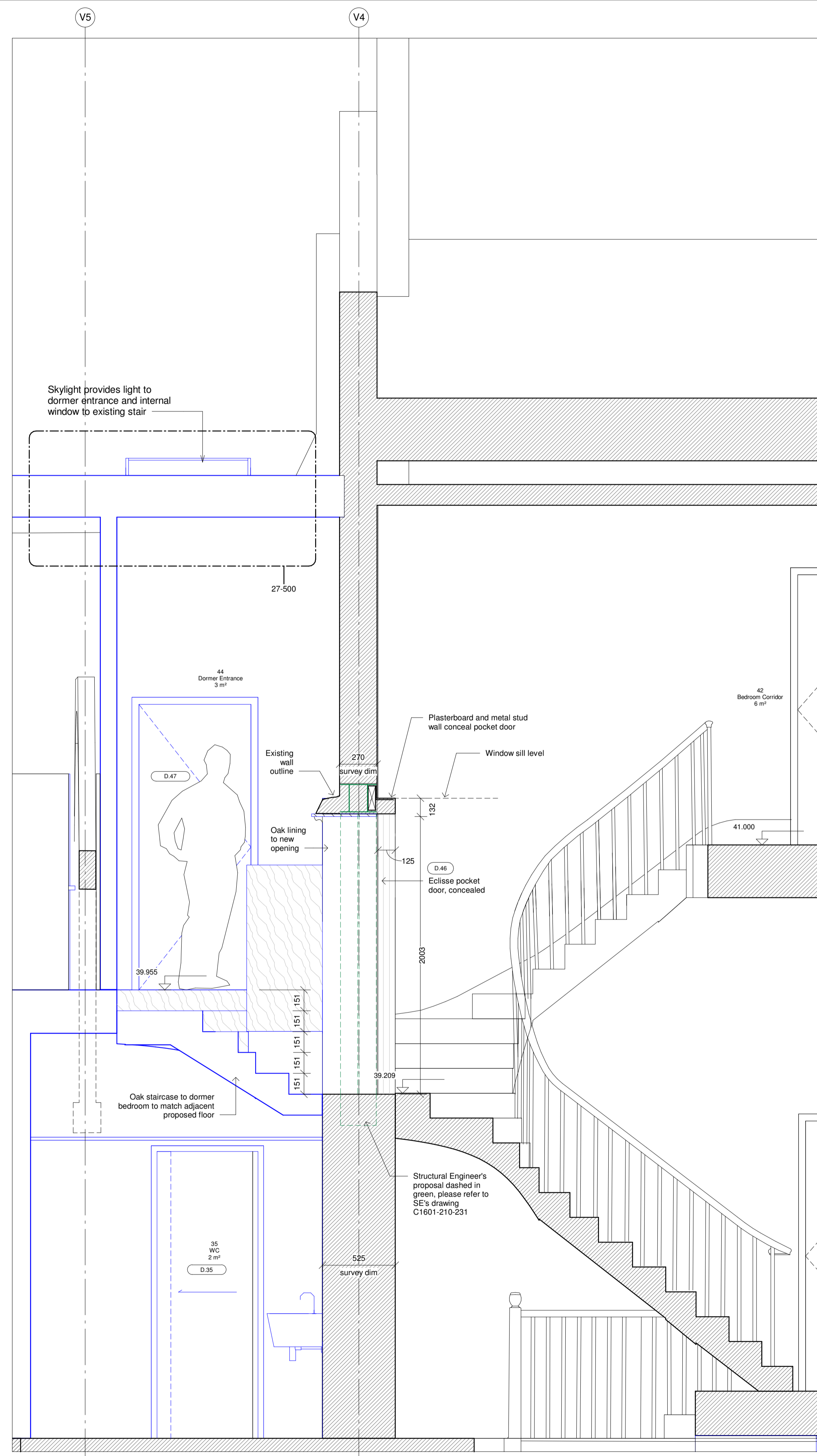
Vicarage - Long Section C.C. 1:20
