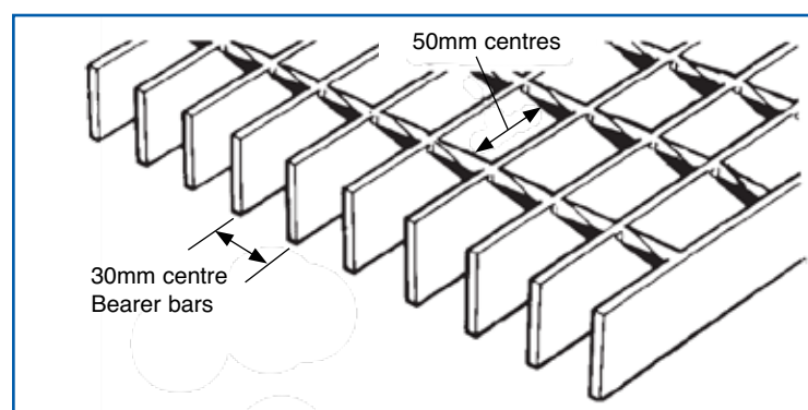
TYPE N50 - 30 / 50
