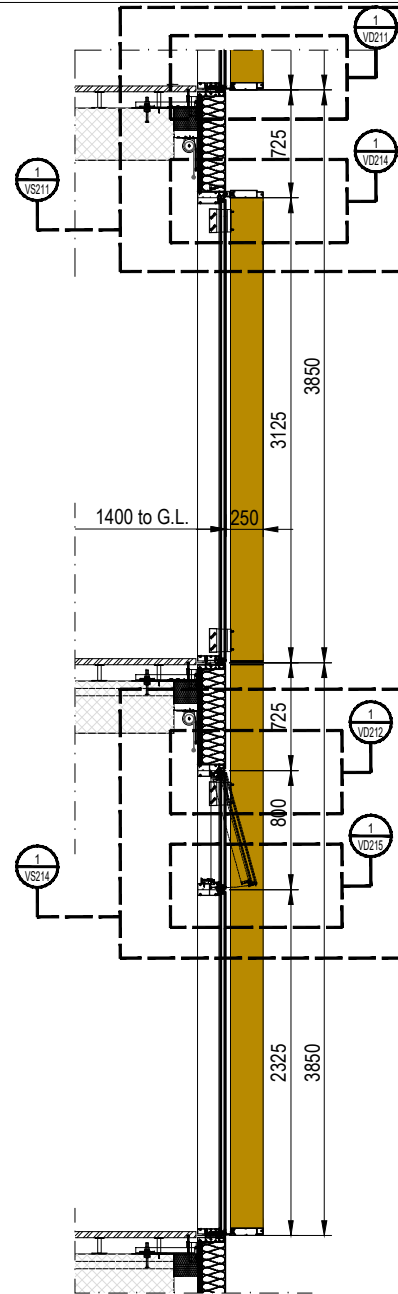
3 Vertical Section Scale: 1:50
