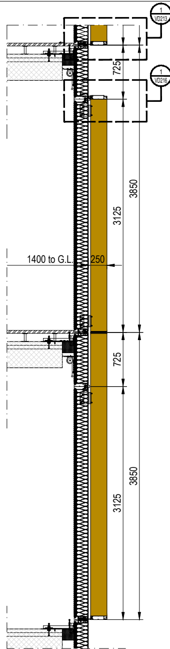
4 Vertical Section Scale: 1:50
