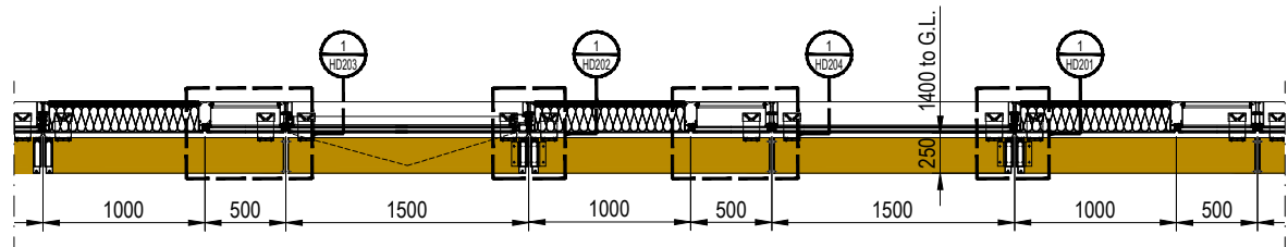
1 Horizontal Section Scale: 1:50
