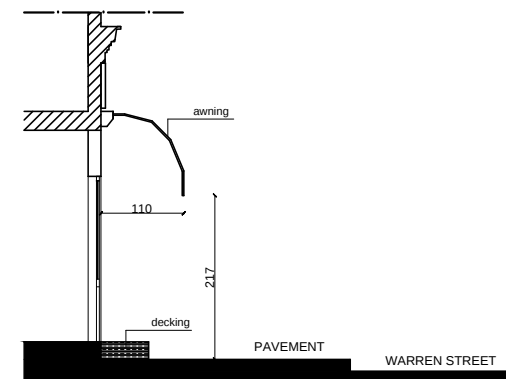
EXISTING SECTION AA SCALE: 1/100 @ A3
