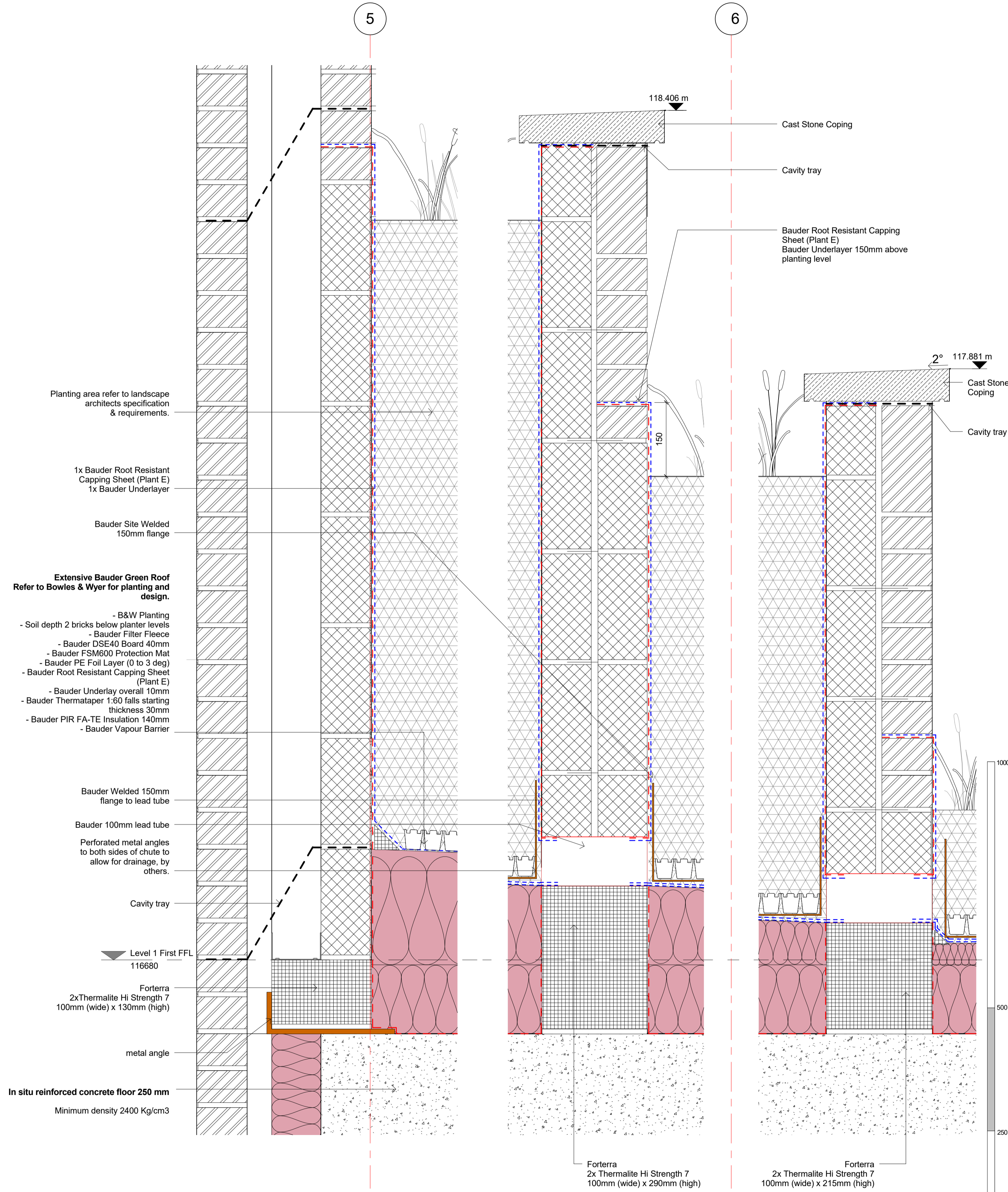
Section F - Planter 2 1 : 5
