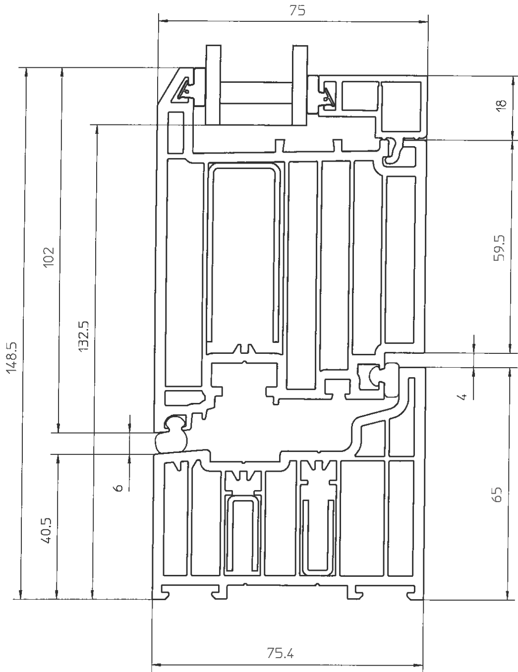
R7002 Frame - 27 Outer R003FD Sash - Flush Door Sash
