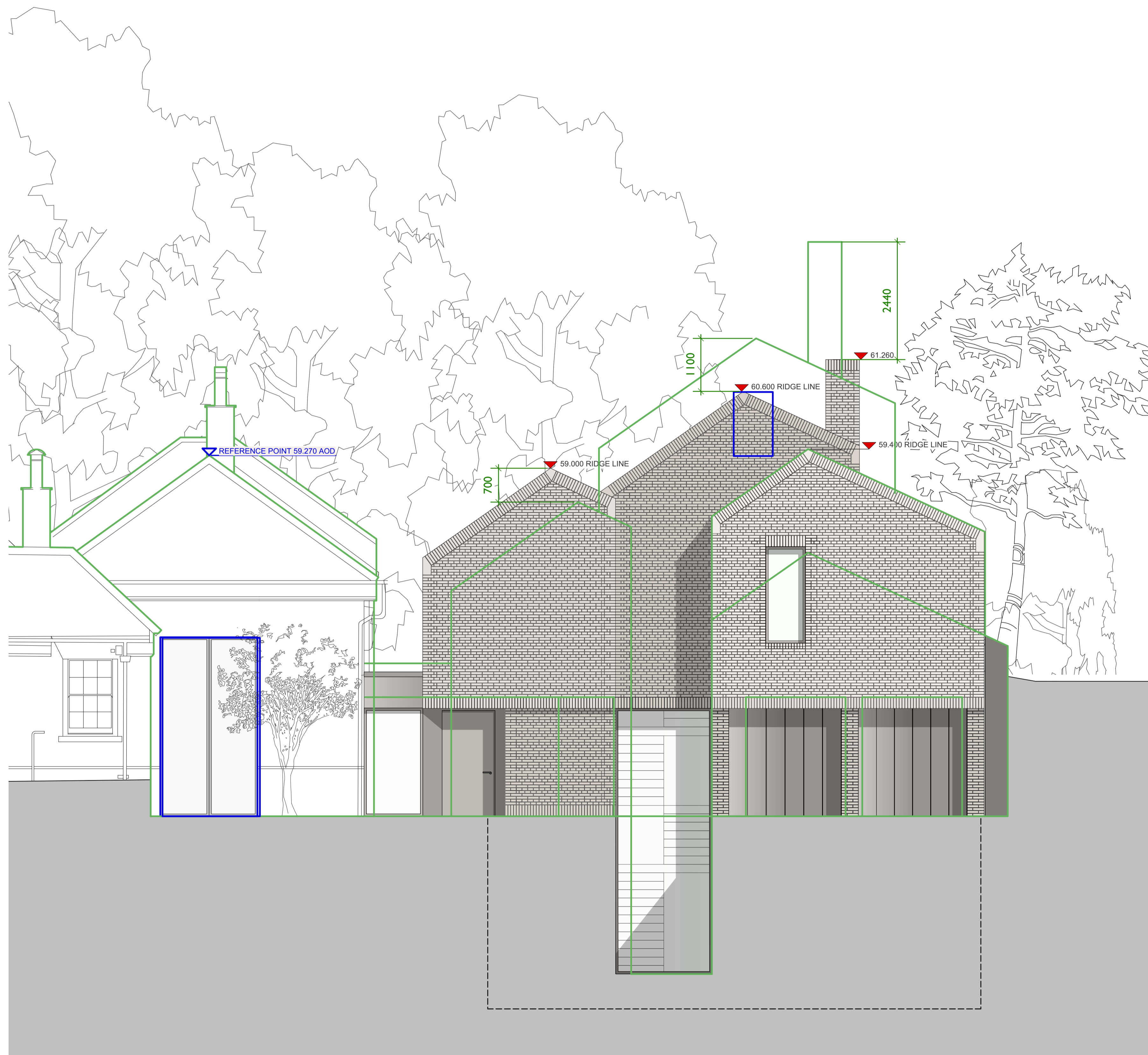
SECTION A-A
