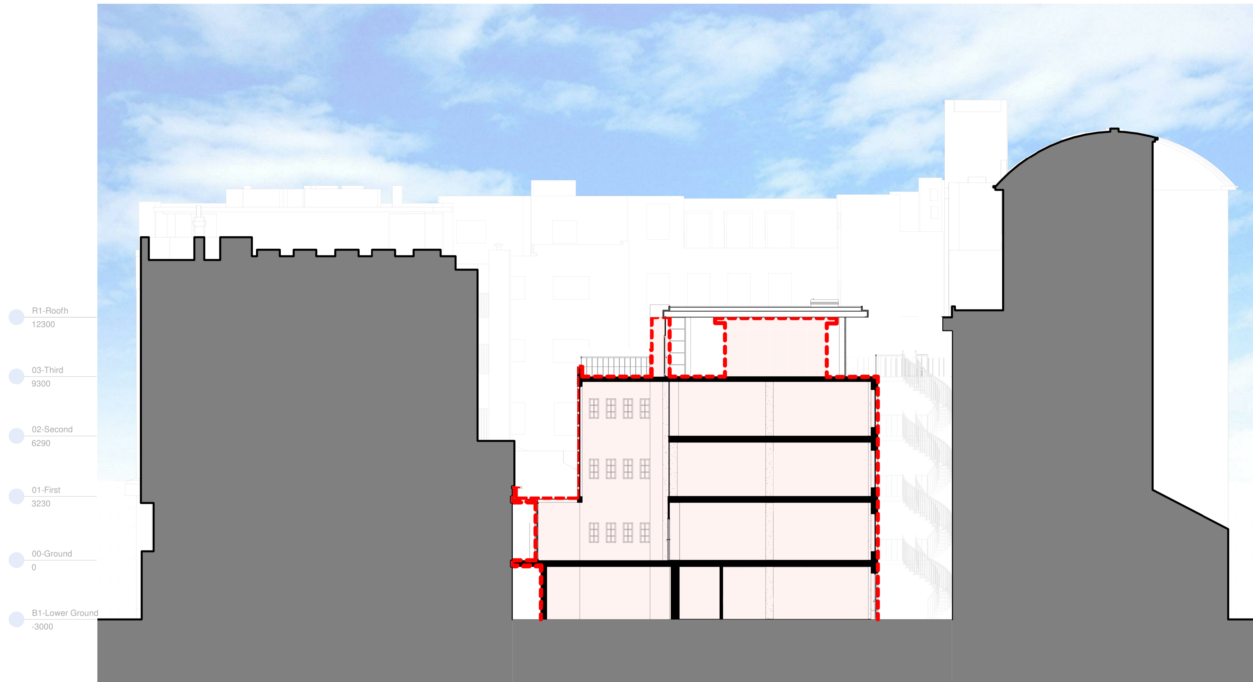
BB Section BB 1 : 100
