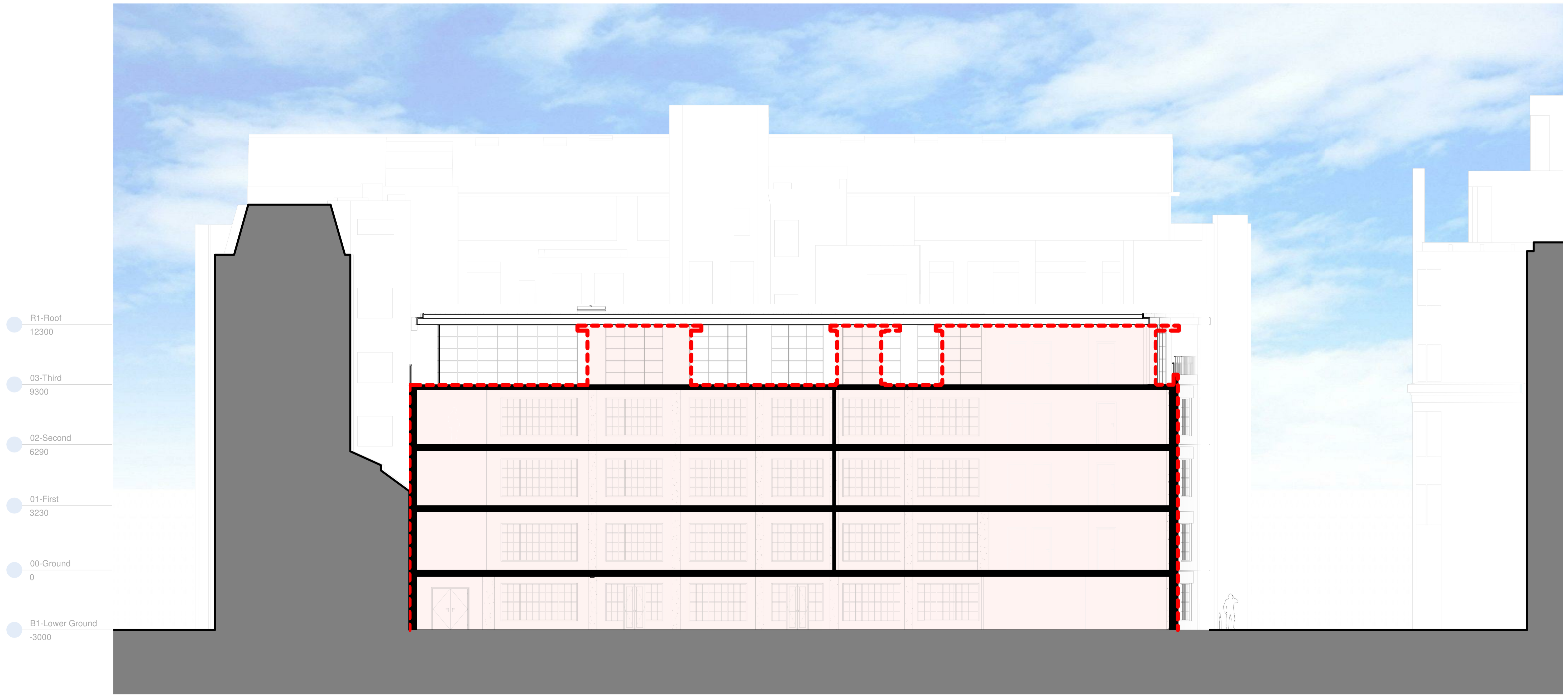
AA Section AA 1 : 100
