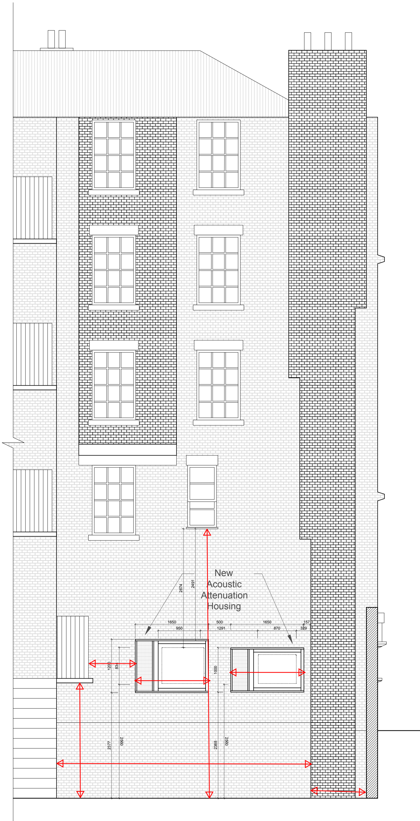
1 Elevation 1:50 @ A3
