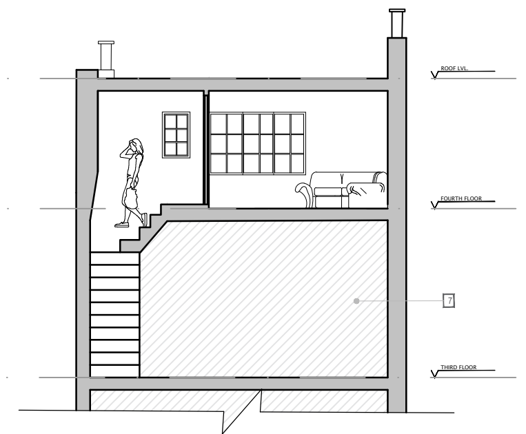
8 SECTION DD EXISTING 1:100
