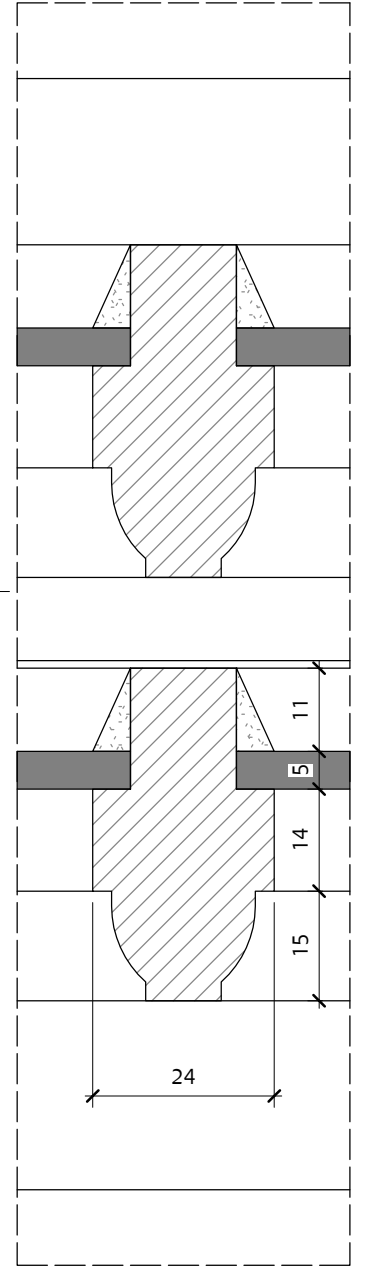
04 Detail 04 1 : 1
