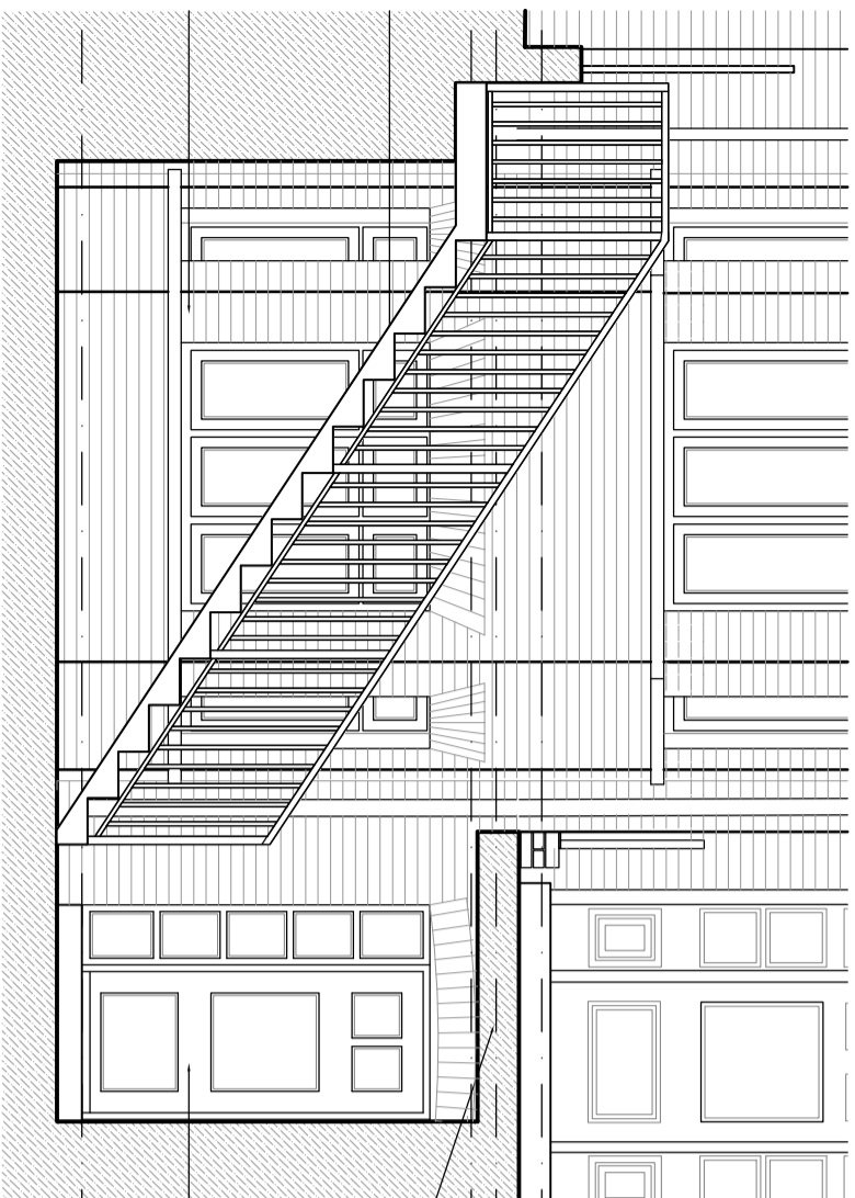
Section A-A
