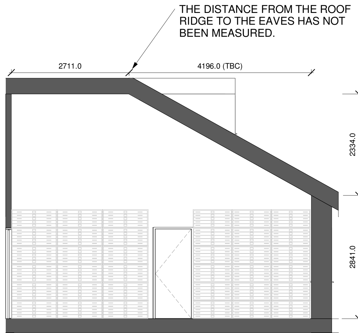
2.2 X18-Elevation 1 : 50
