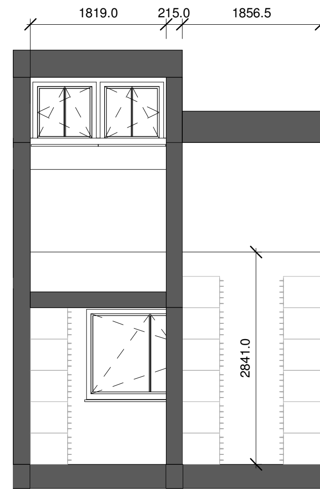
2.3 X18-Elevation 1 : 50
