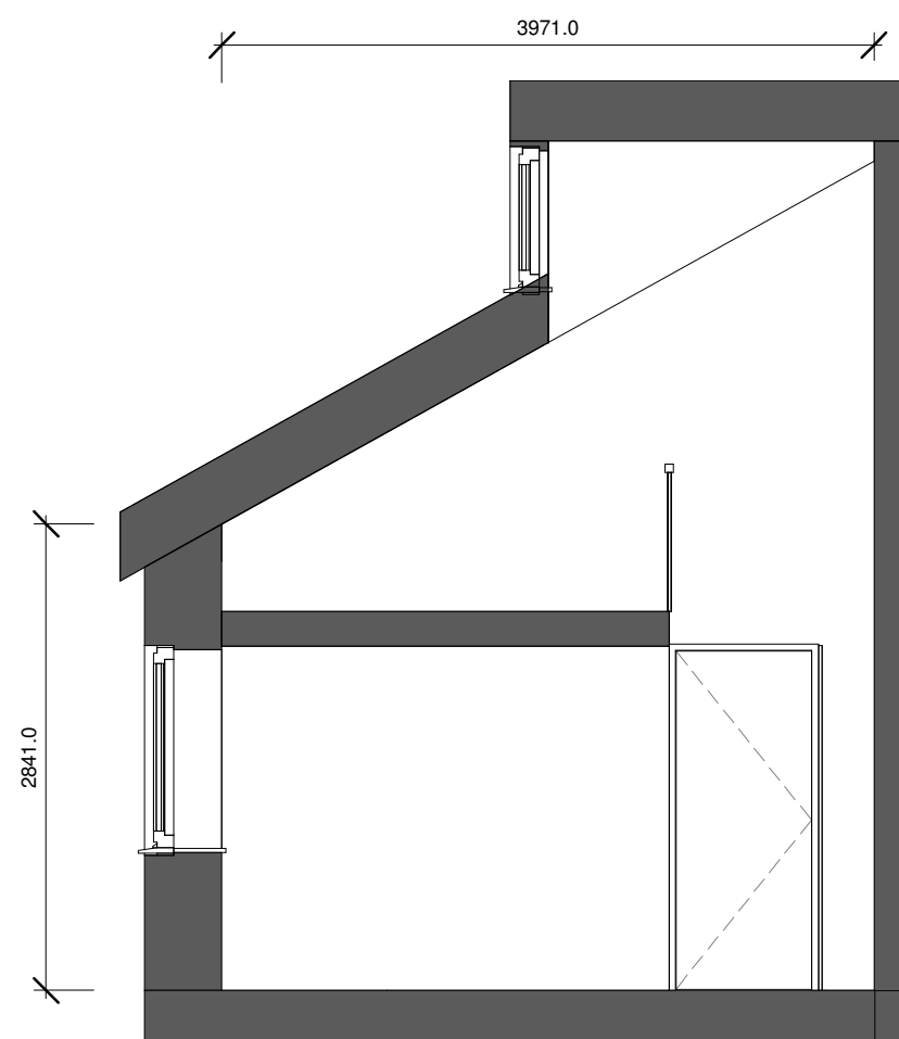
2.7 X18A-Elevation 1 : 50
