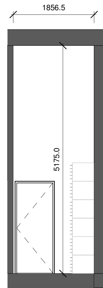
2.1 X18-Elevation 1 : 50
